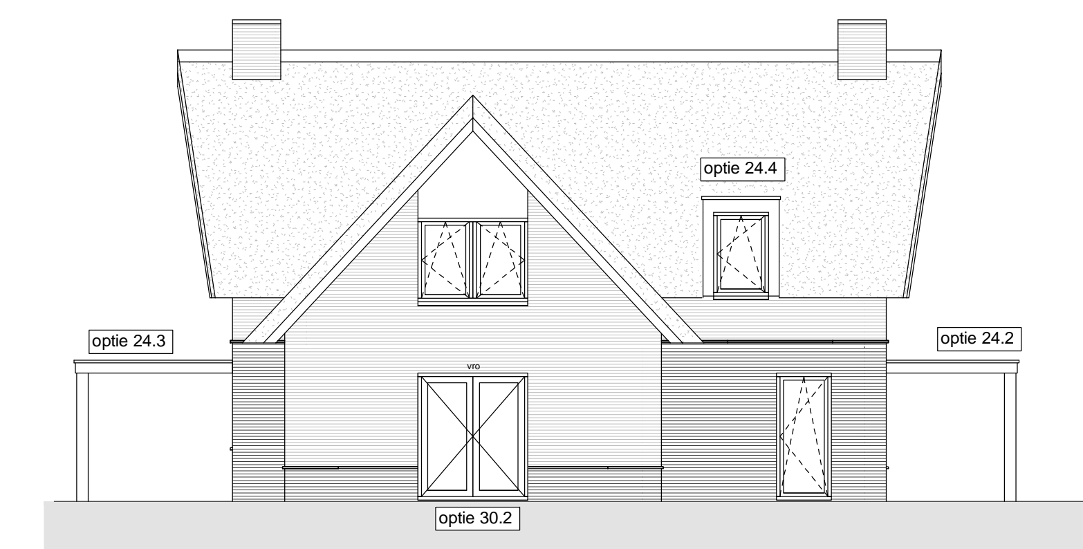
Linkergevel 1 : 100
