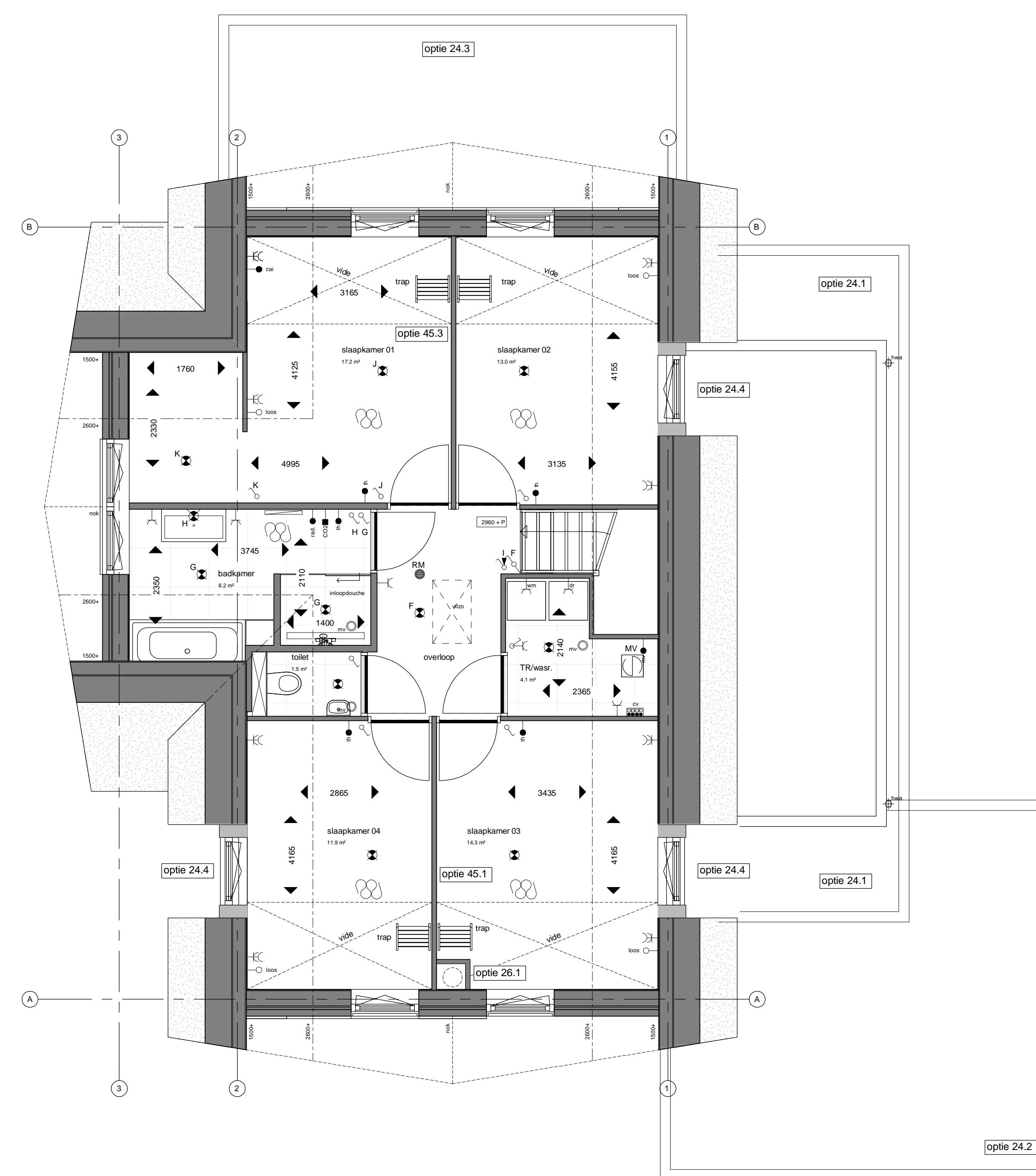
Eerste verdieping type A1 1 : 50
