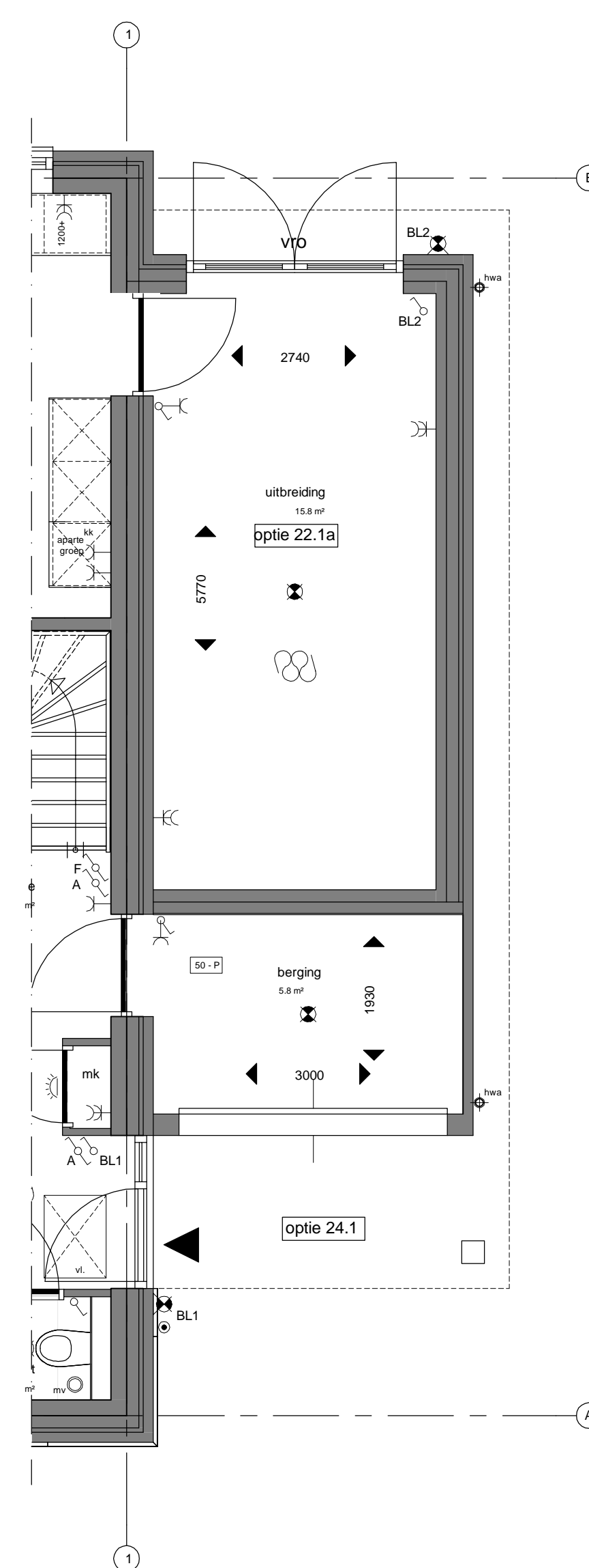
Fragment Begane grond type A1 Bouwnummers 12 en 20 1 : 50
