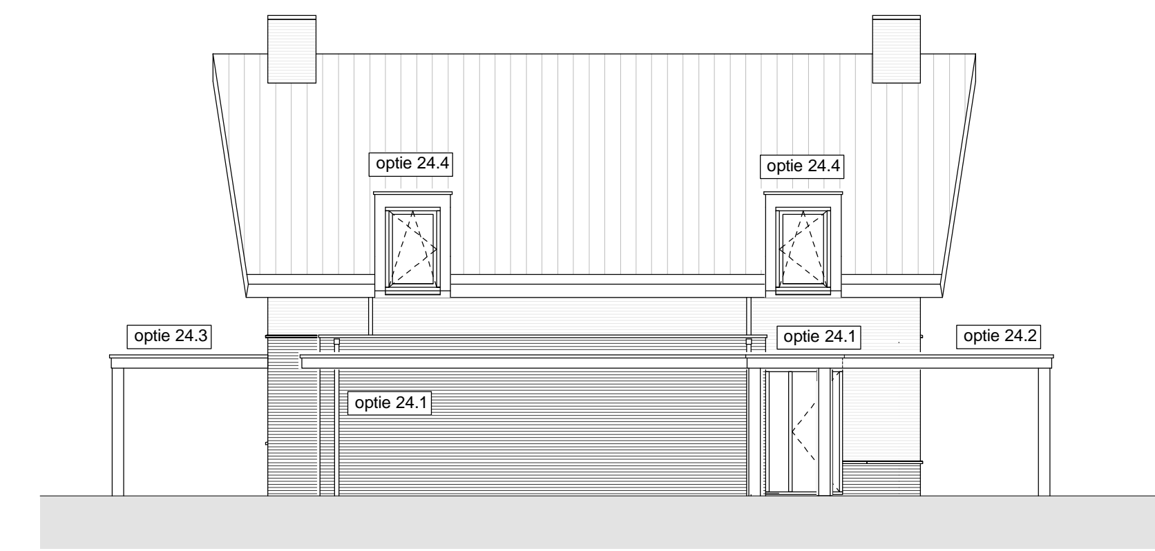
Linkergevel 1 : 100
