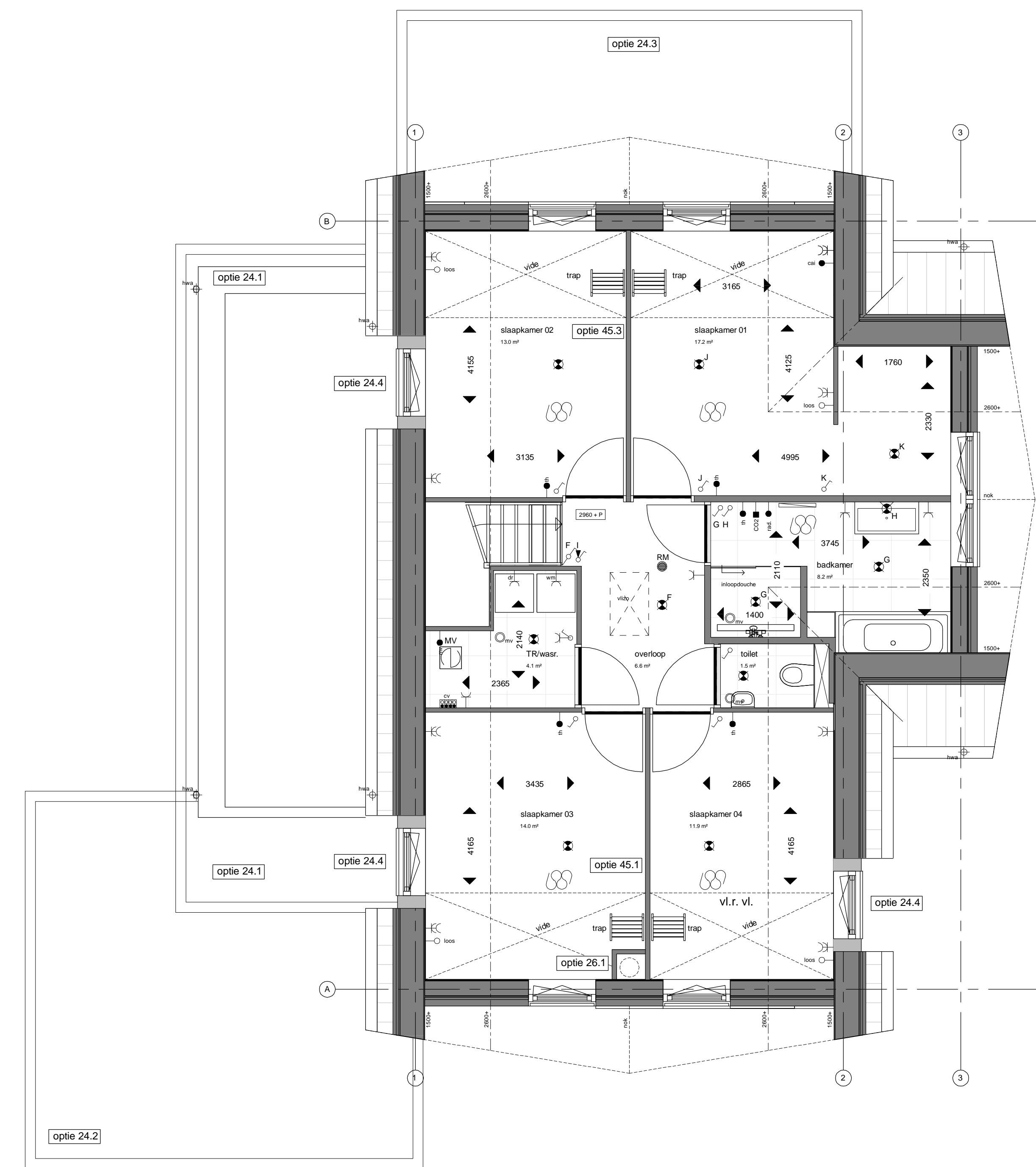
Eerste verdieping type A 1 : 50
