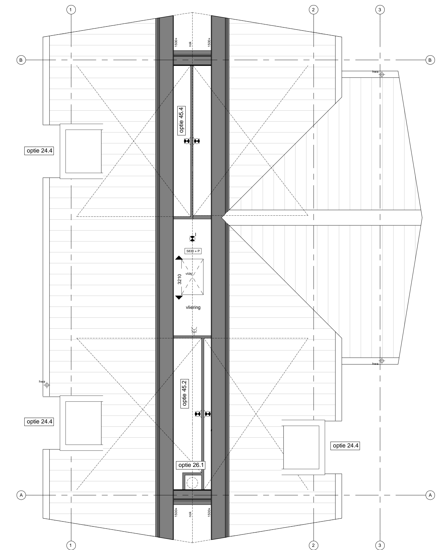
Vliering type A 1 : 50
