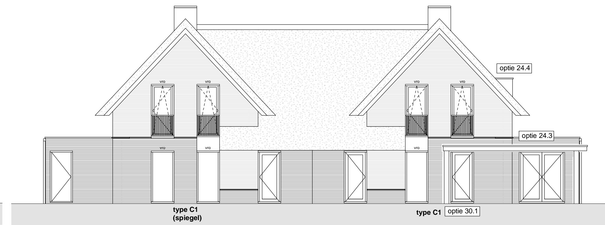
Achtergevel 1 : 100
