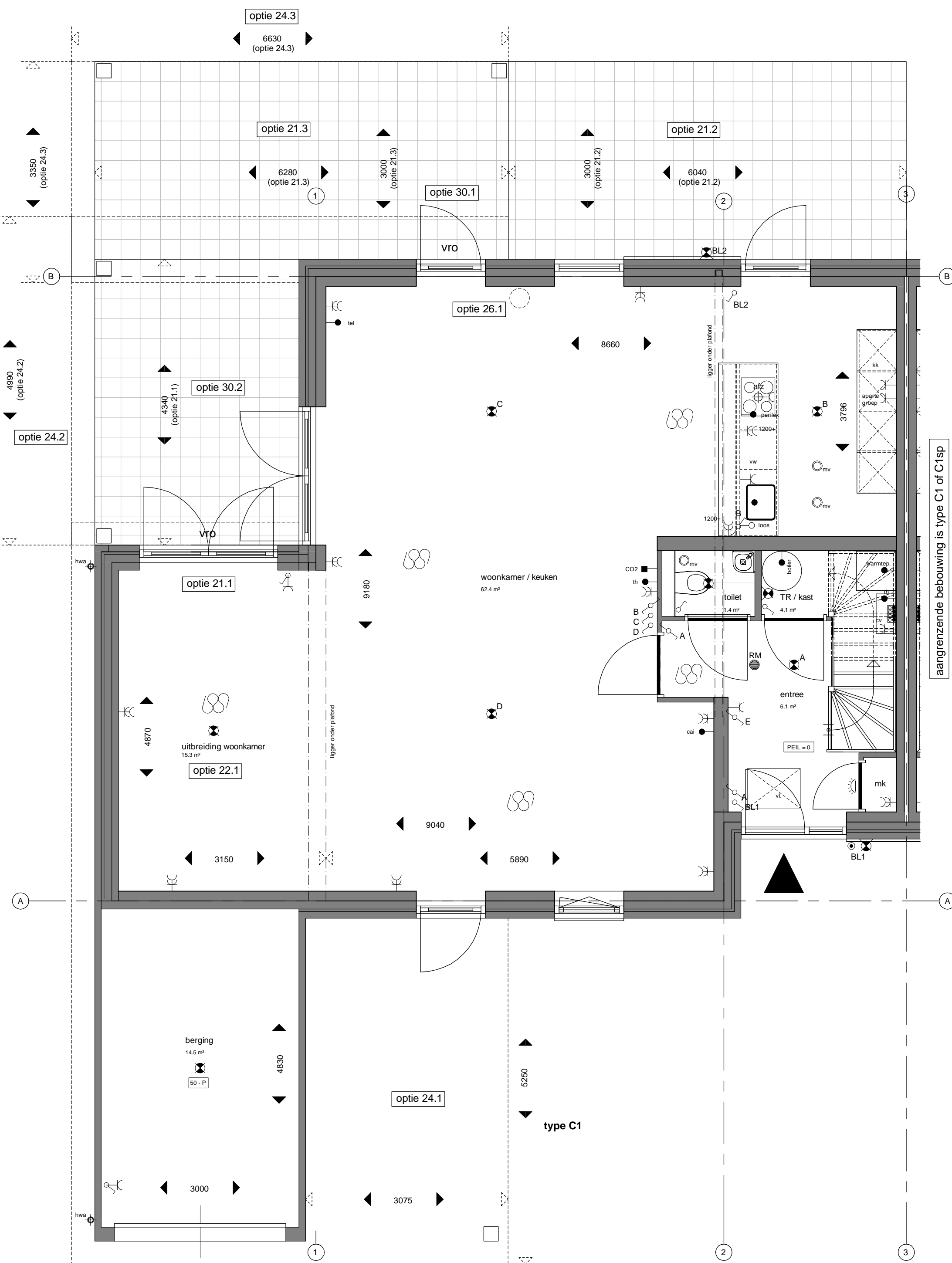
Begane grond type C1 Bouwnummer 3 en 8 Bouwnummer gespiegeld 2 en 7 1 : 50
