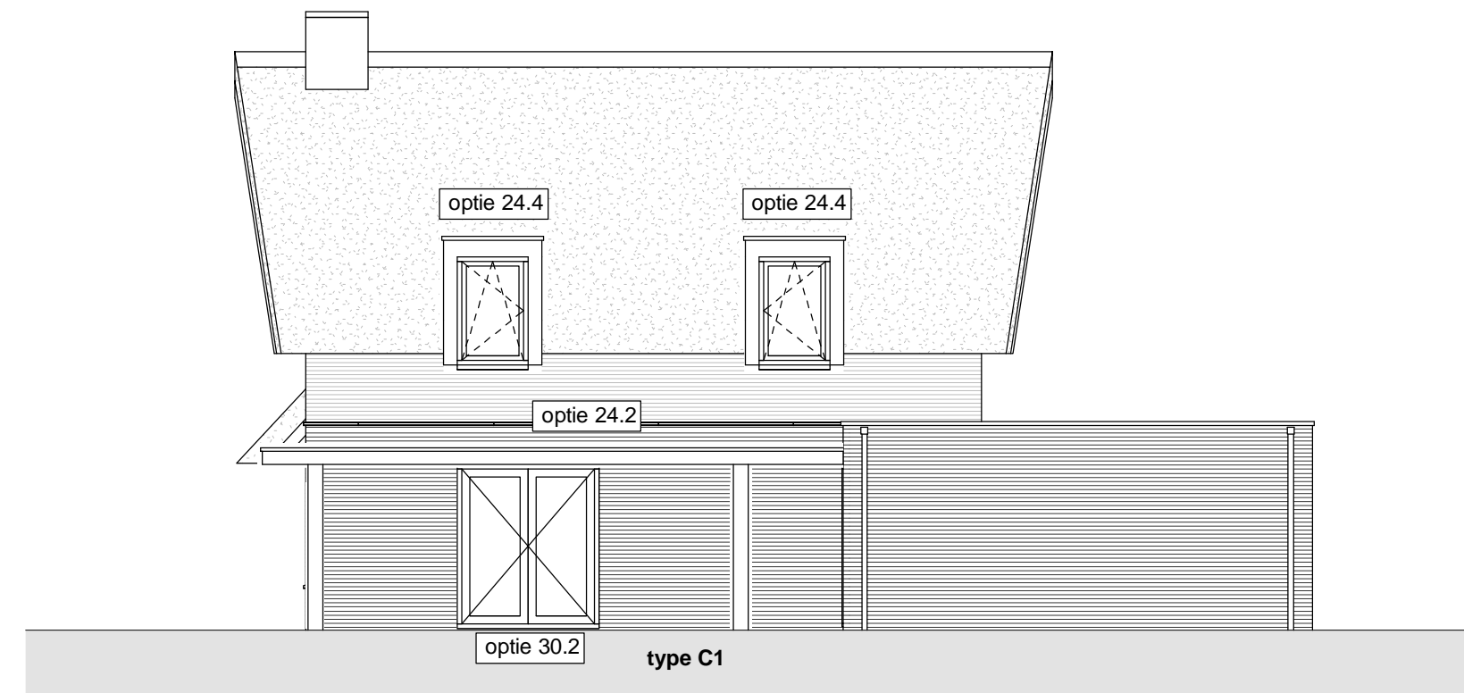
Linkergevel 1 : 100
