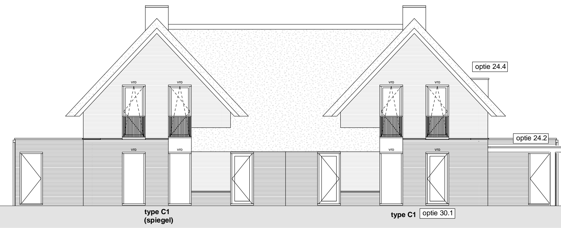
Achtergevel 1 : 100
