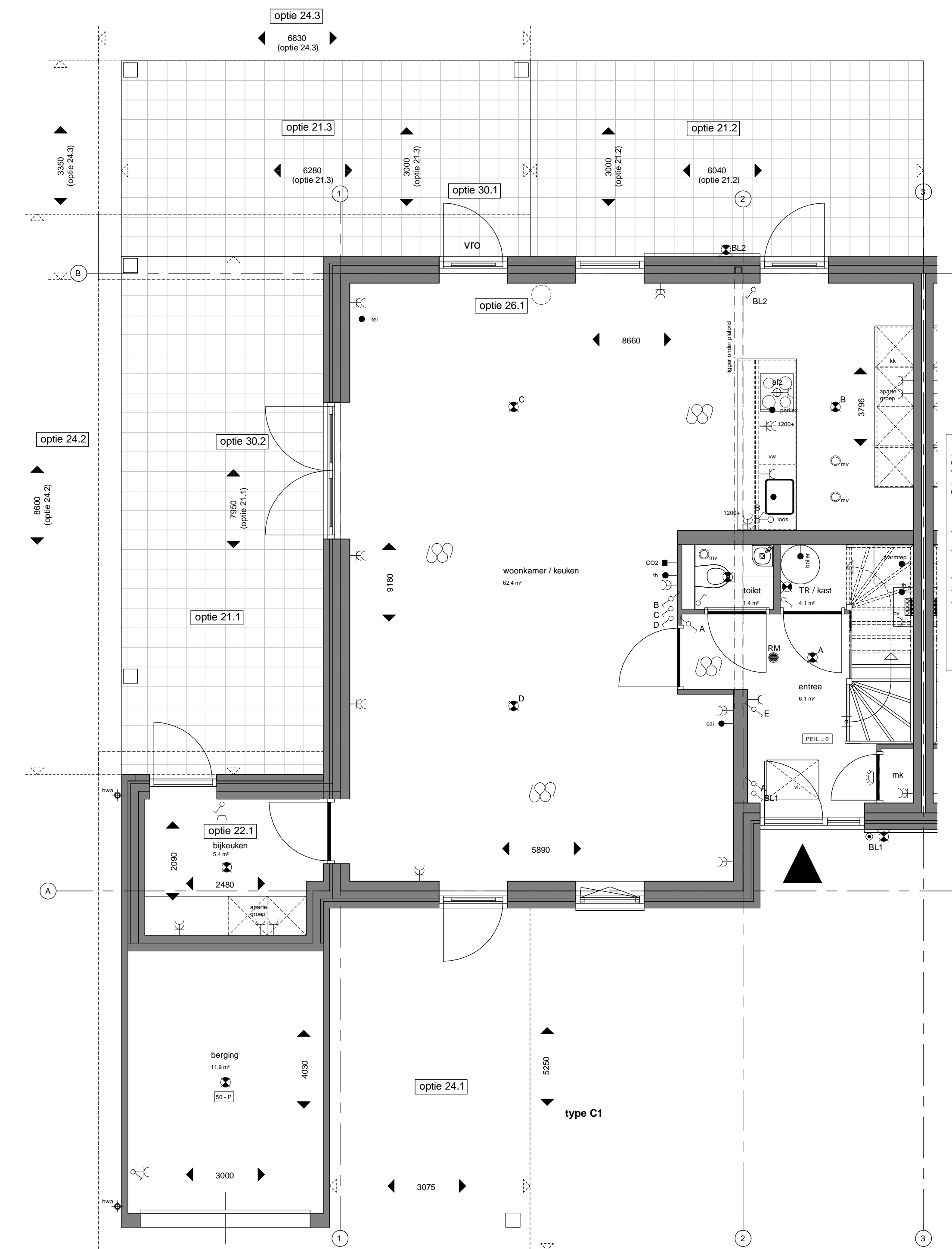
Begane grond type C1 Bouwnummer 3 en 8 Bouwnummer gespiegeld 2 en 7 1 : 50
