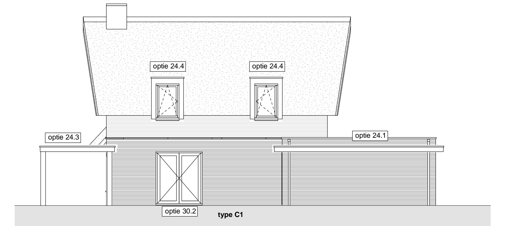
Linkergevel 1 : 100
