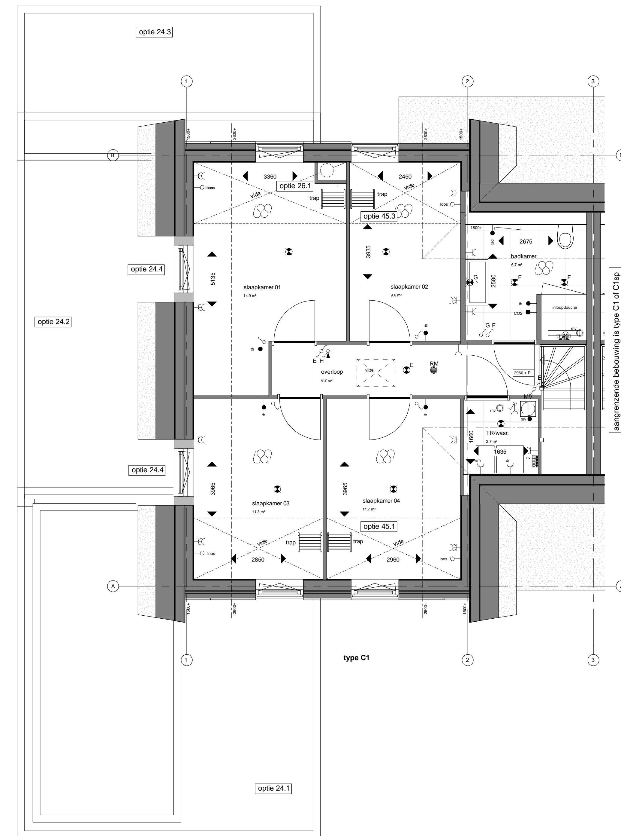
Eerste verdieping type C1 1 : 50
