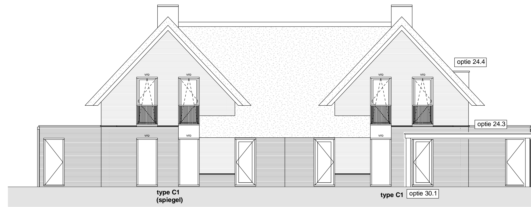
Achtergevel 1 : 100
