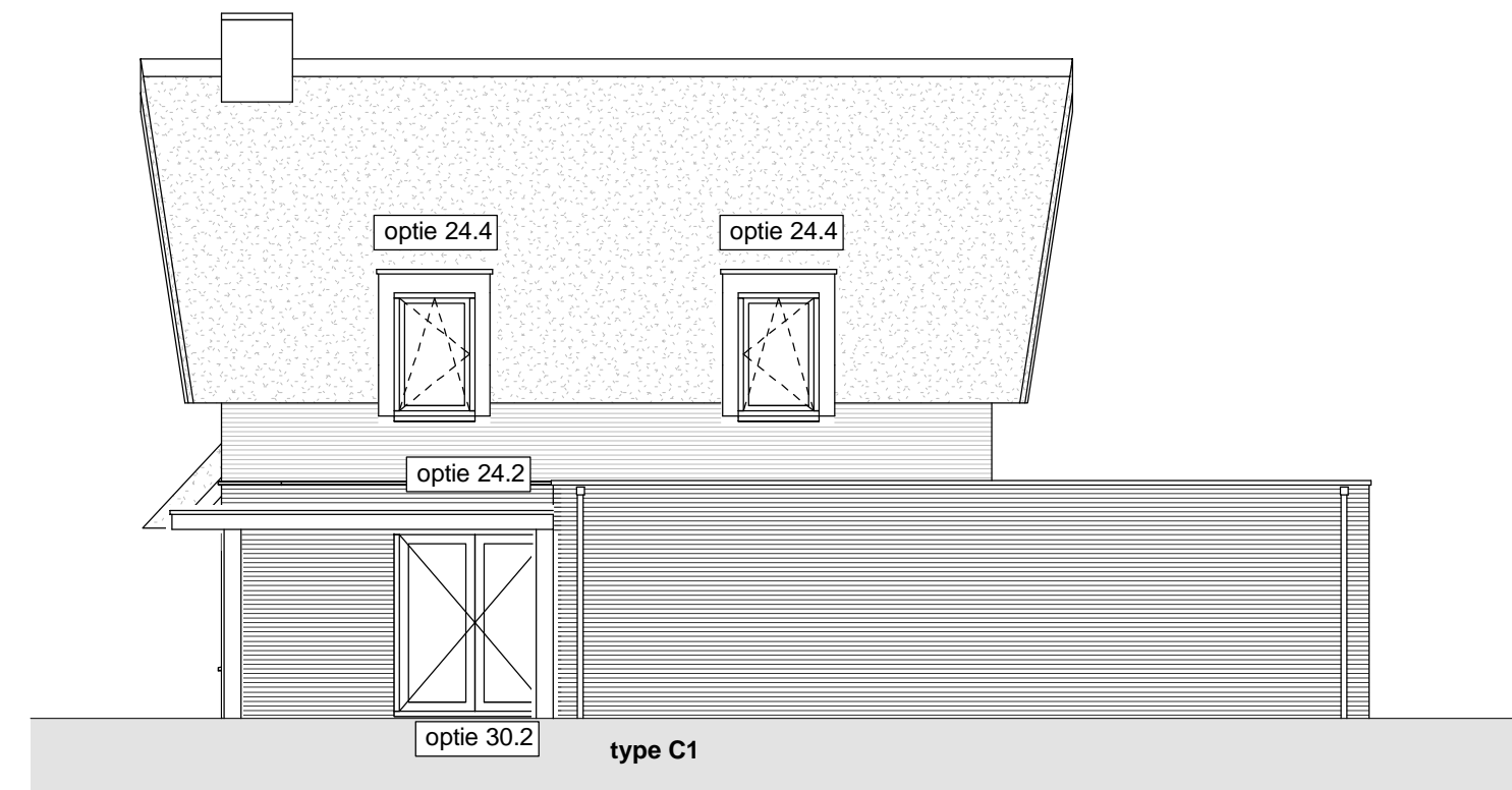
Linkergevel 1 : 100
