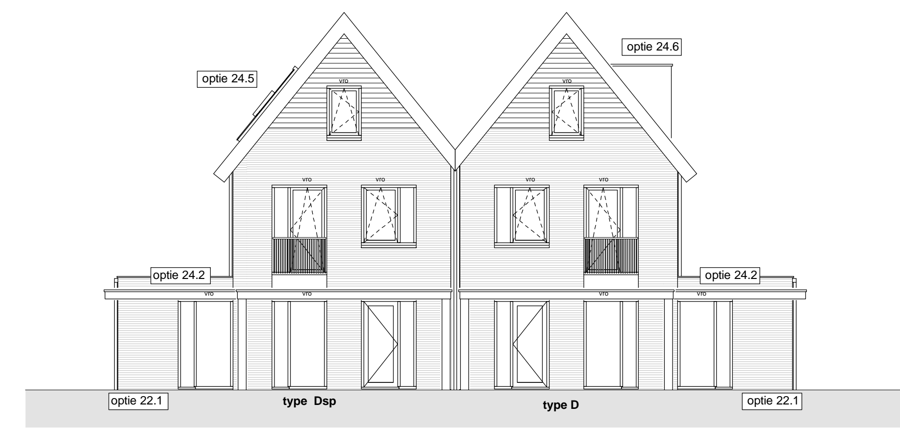
Achtergevel
