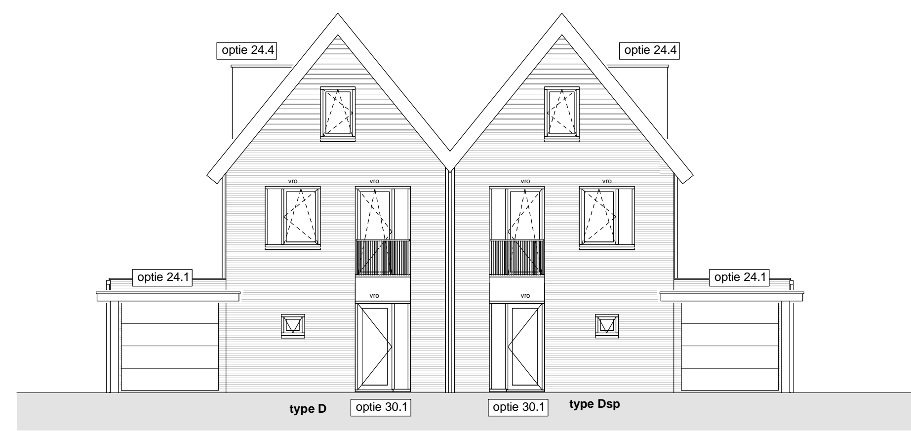
Voorgevel
