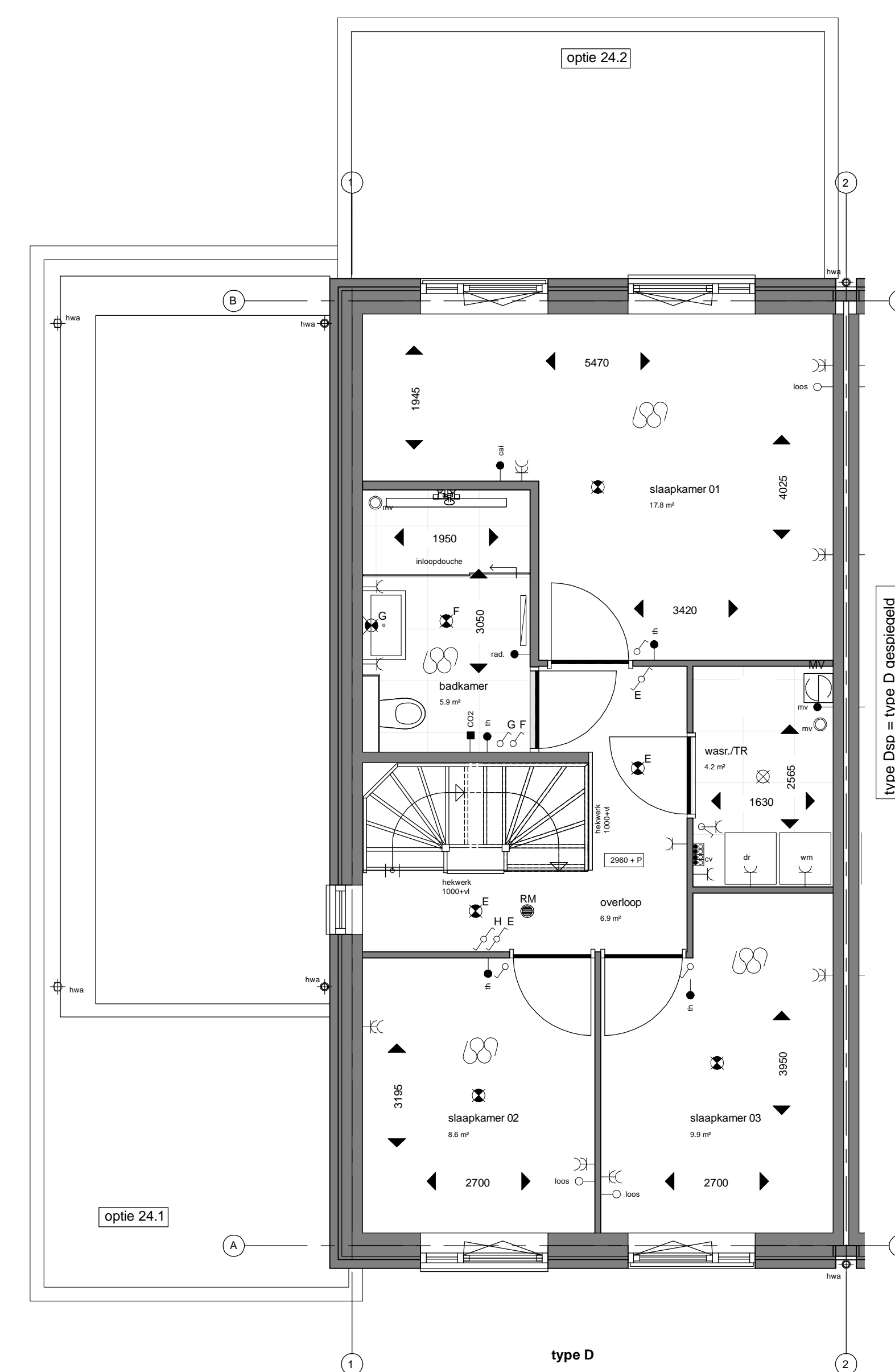
Eerste verdieping type D
