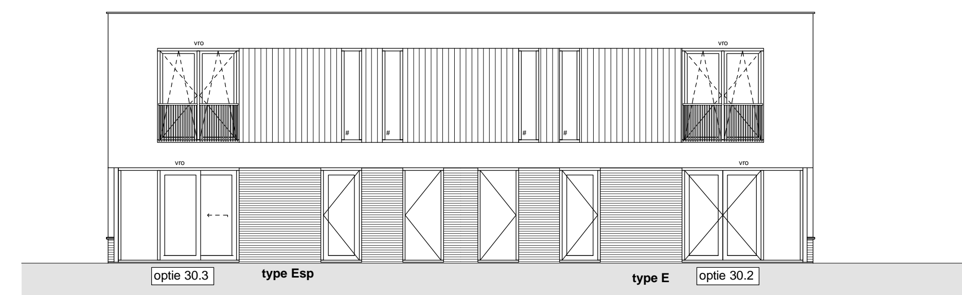
Achtergevel 1 : 100
