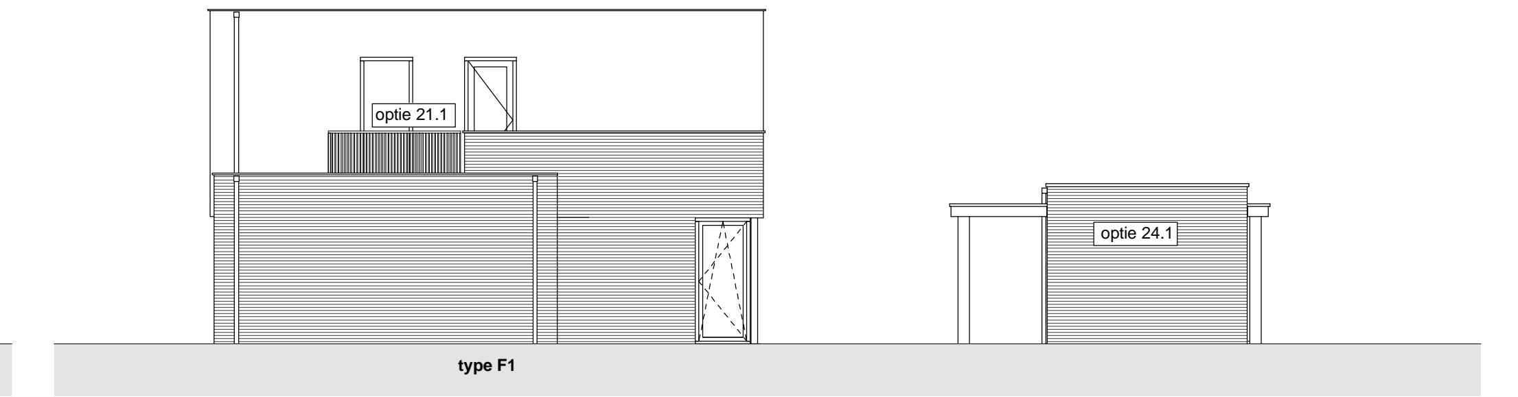
Linkergevel 1 : 100
