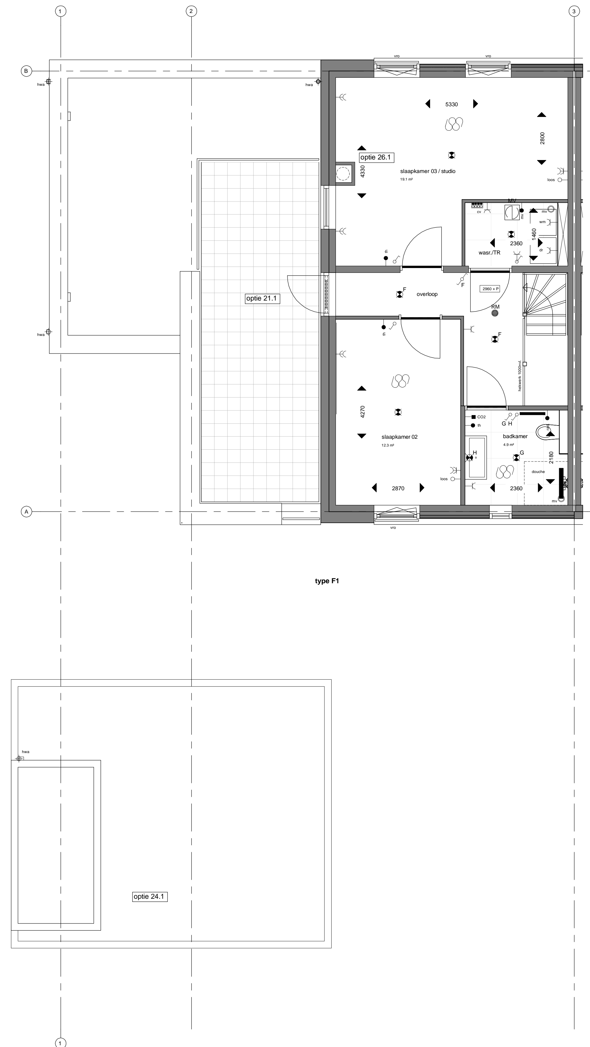
Eerste verdieping type F1 1 : 50
