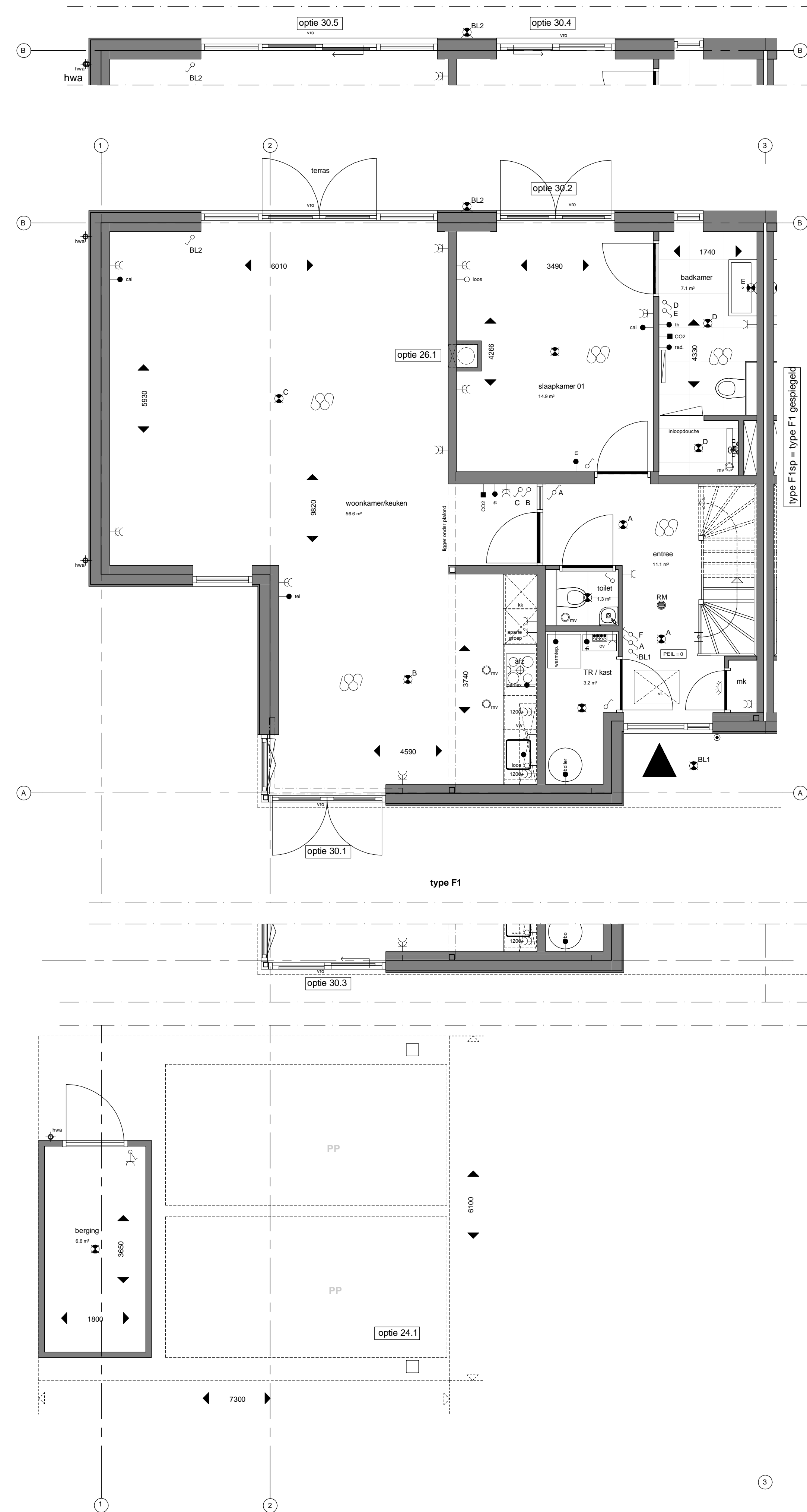
Begane grond type F1 Bouwnummer 14 Bouwnummer gespiegeld 13 1 : 50
