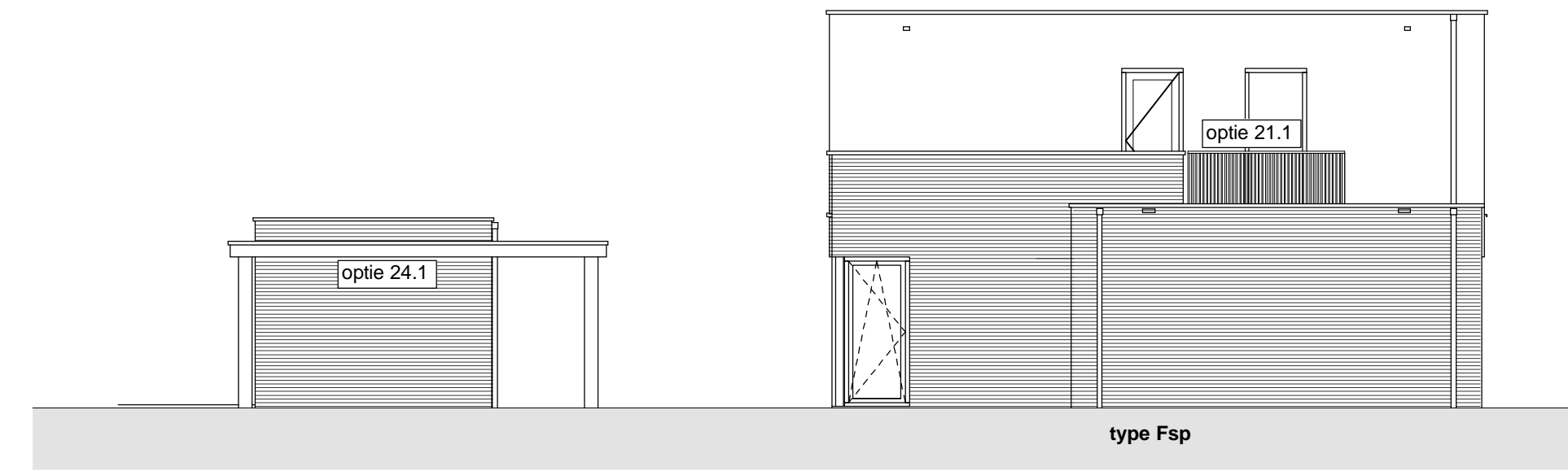
Rechtergevel 1 : 100
