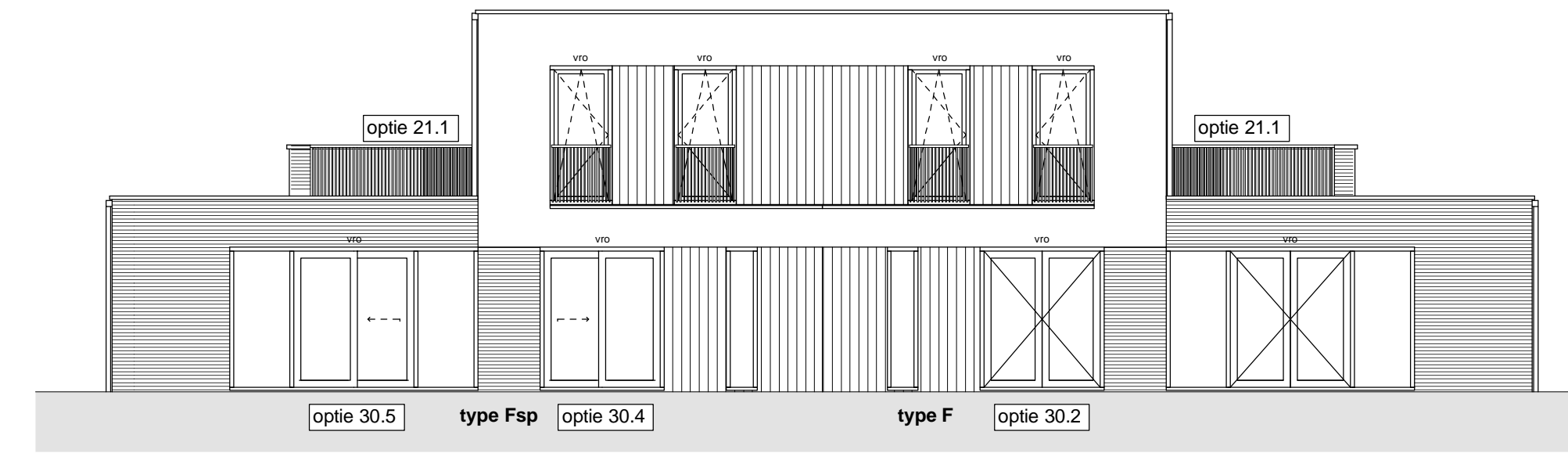
Achtergevel 1 : 100
