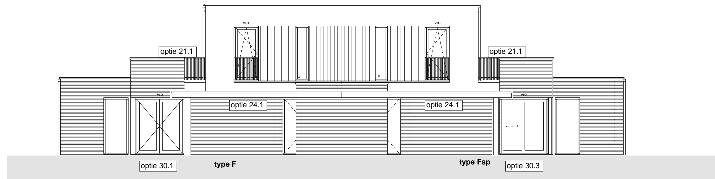
Voorgevel 1 : 100
