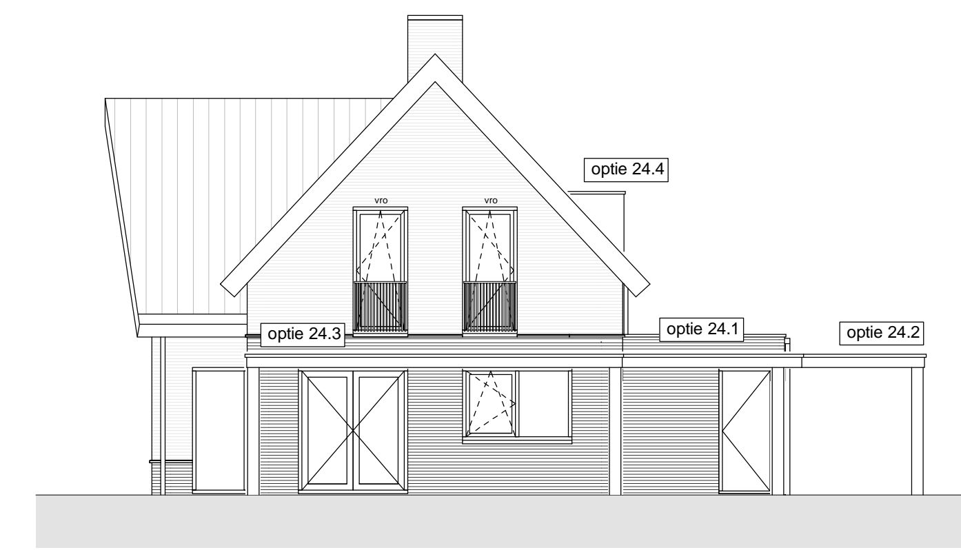
Achtergevel 1 : 100
