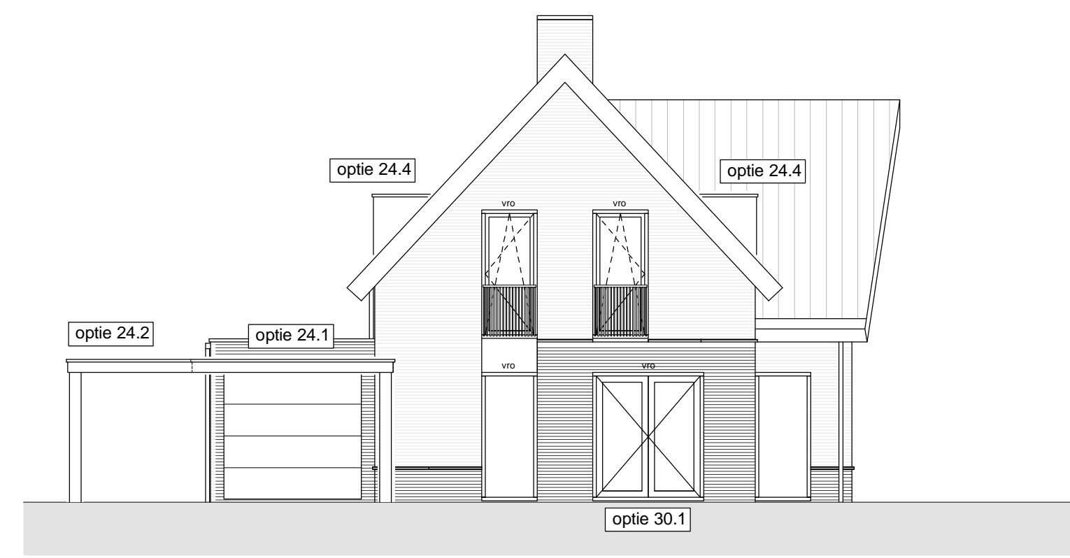
Voorgevel 1 : 100
