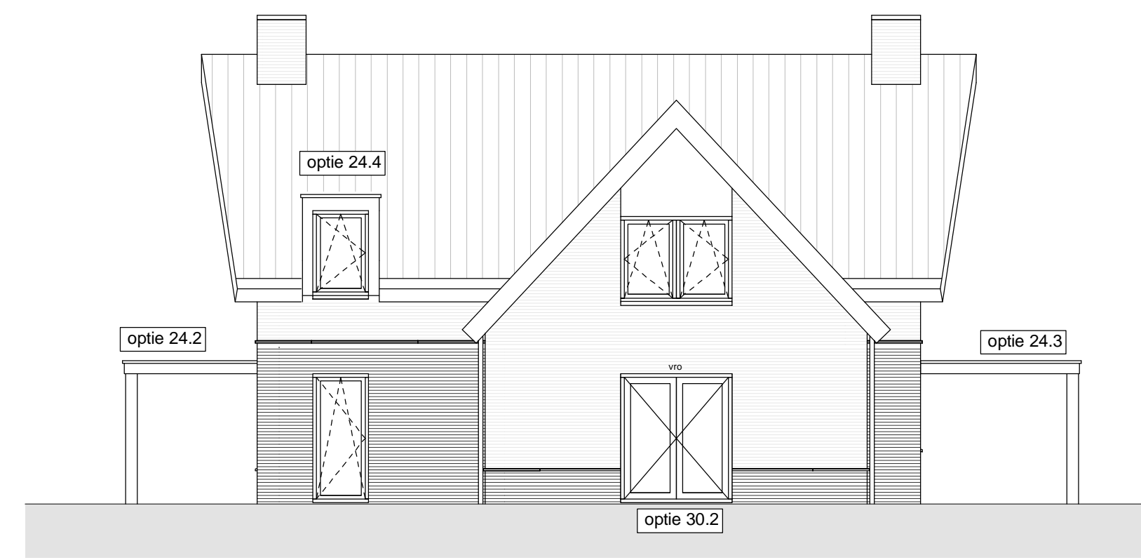
Rechtergevel 1 : 100
