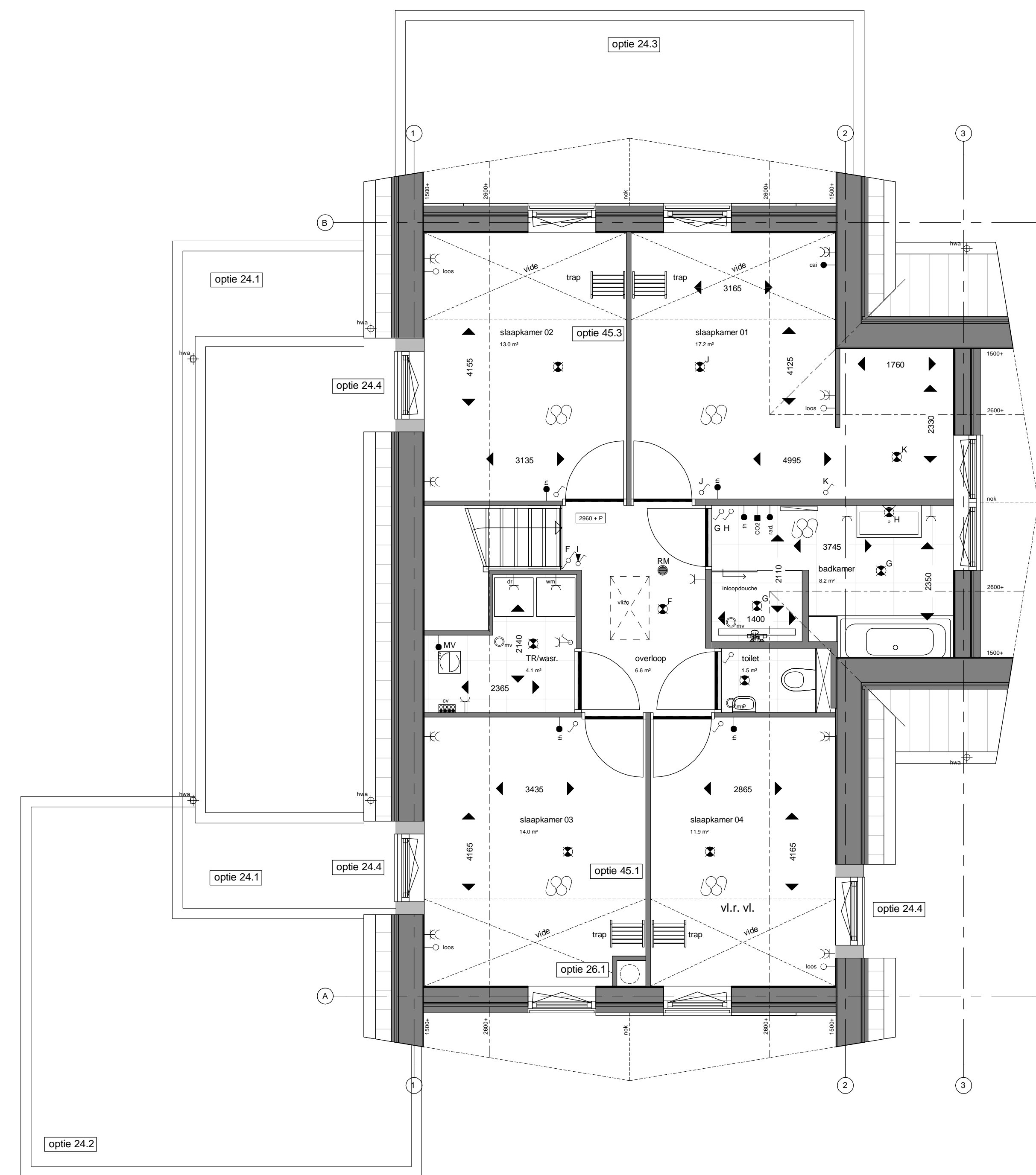
Eerste verdieping type A 1 : 50
