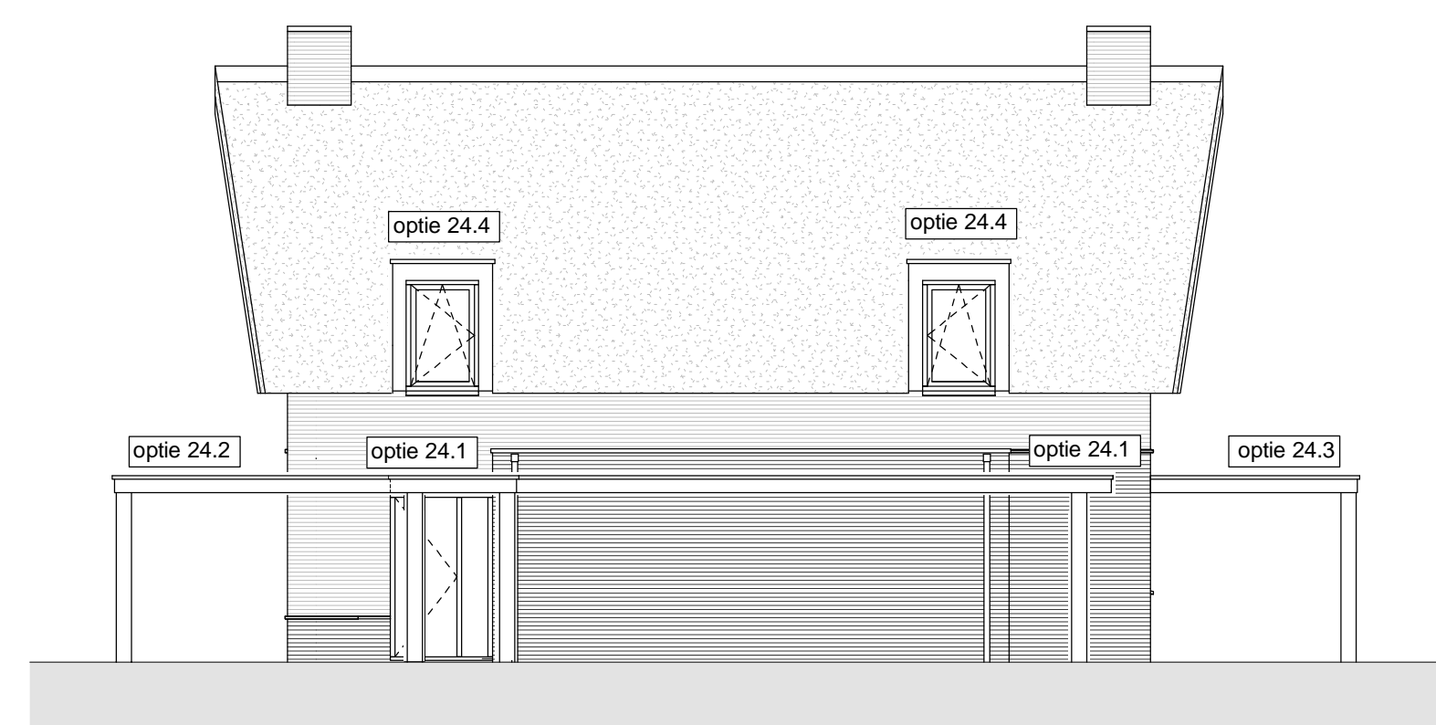
Rechtsgevel 1 : 100
