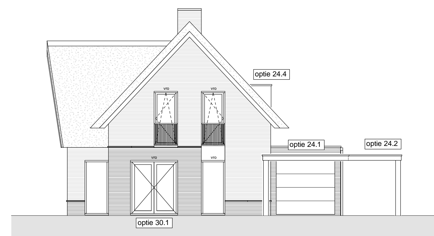
Voorgevel 1 : 100
