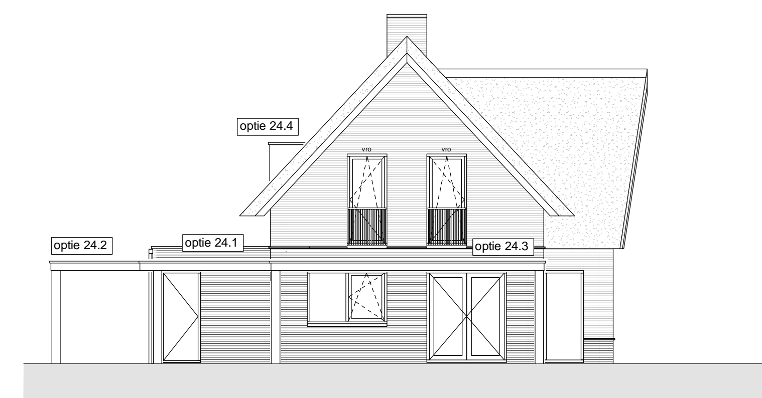
Achtergevel 1 : 100
