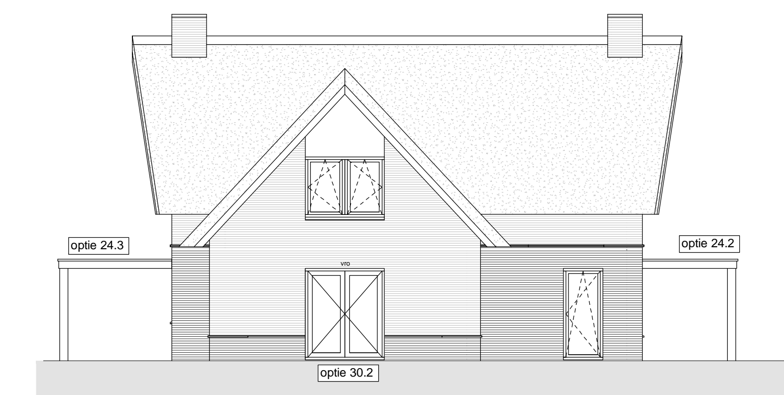
Linkergevel 1 : 100
