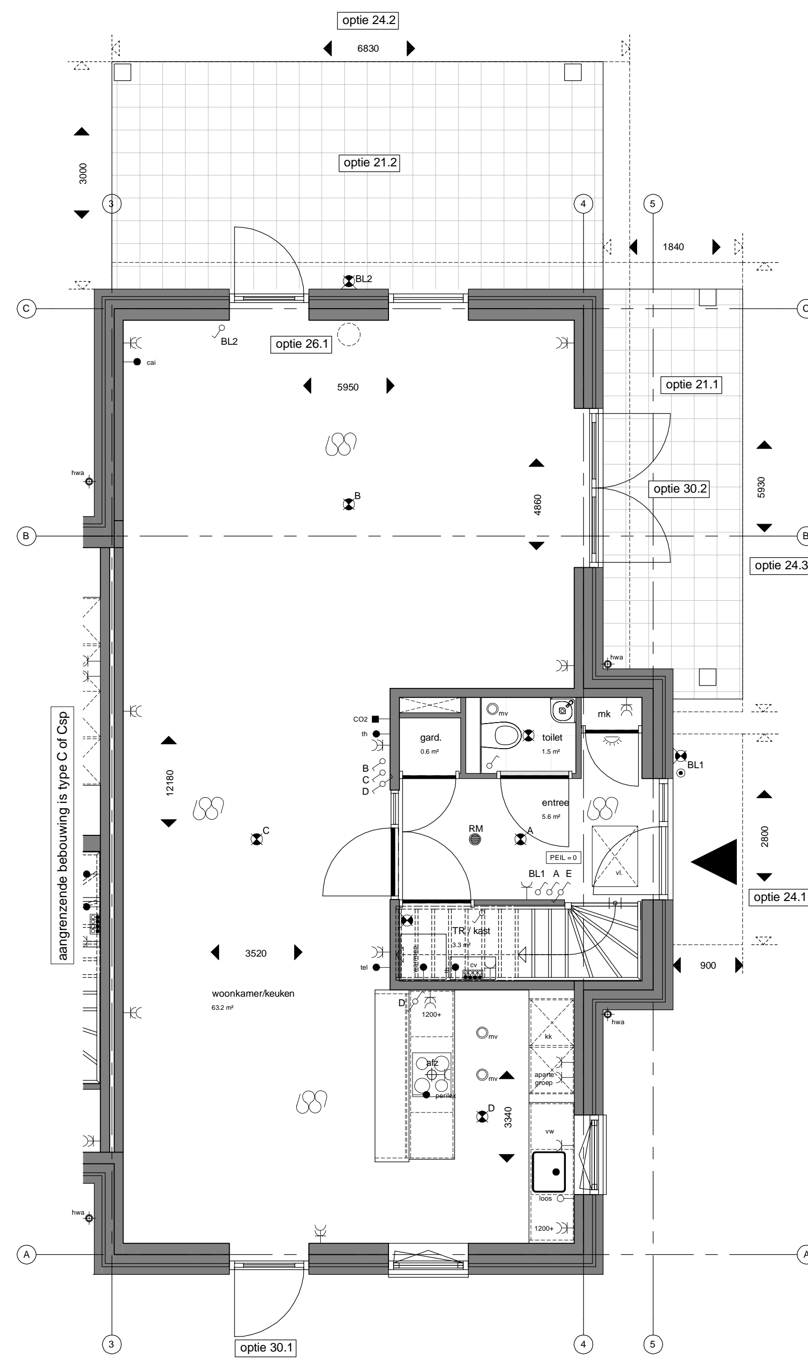
Begane grond type B Bouwnummer 11 Bouwnummer gespiegeld 10 1 : 50
