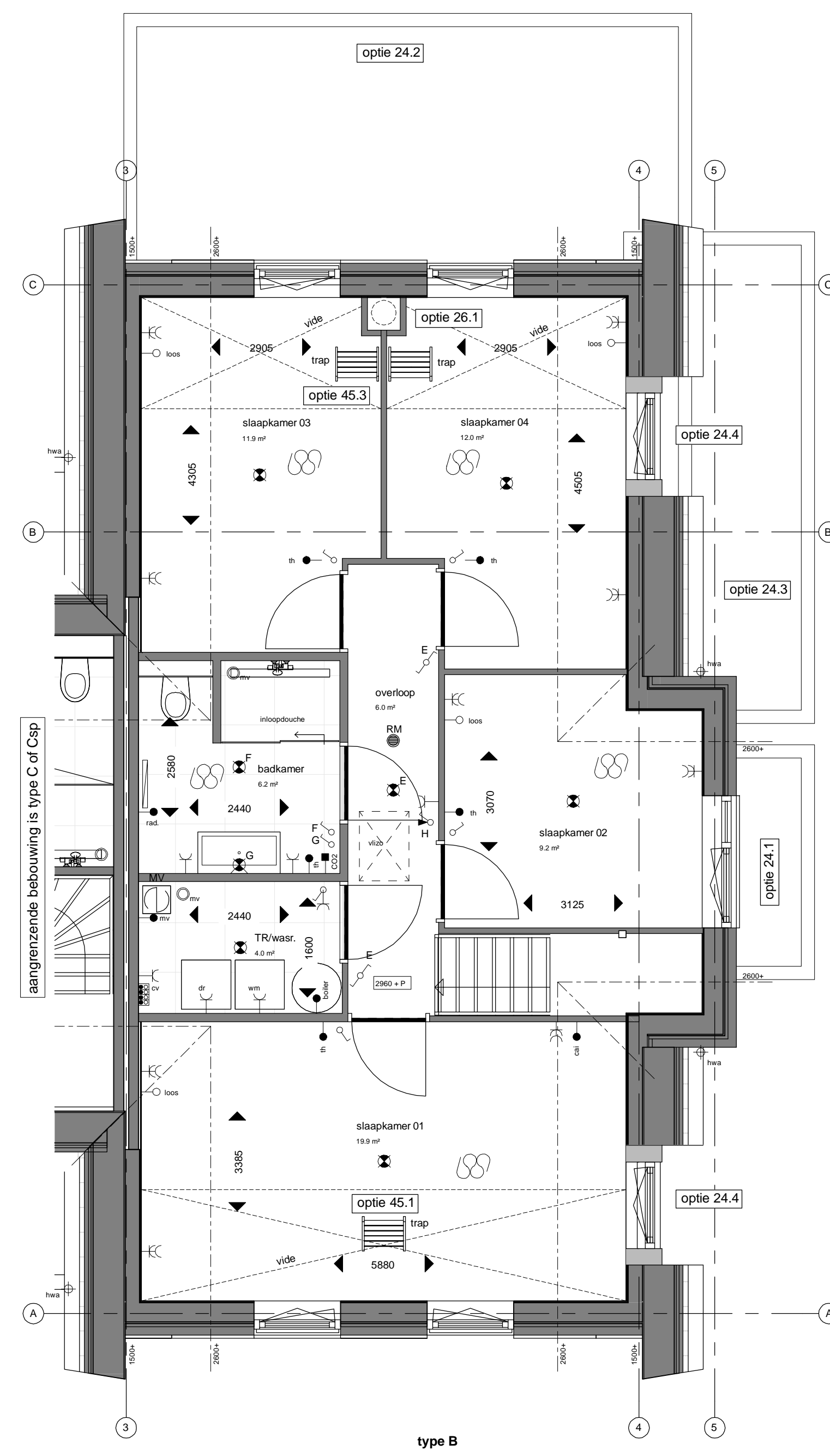
Eerste verdieping type B 1 : 50
