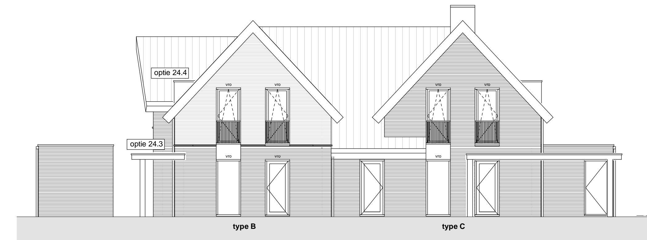
Achtergevel 1 : 100
