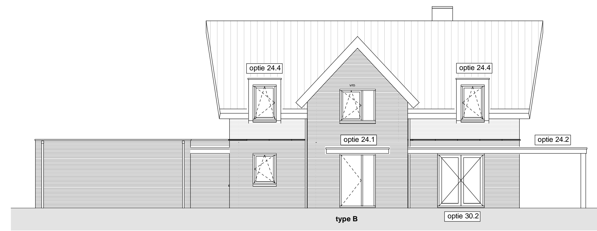
Rechtergevel 1 : 100
