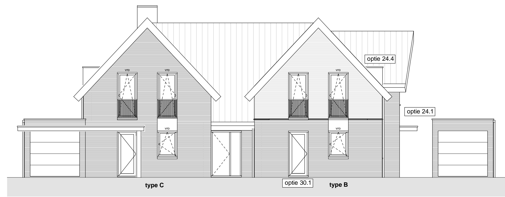
Voorgevel 1 : 100
