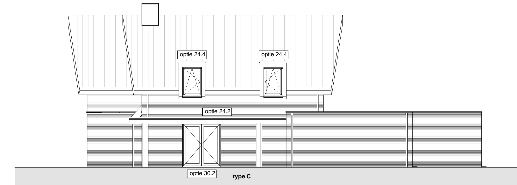
Linkergevel 1 : 100
