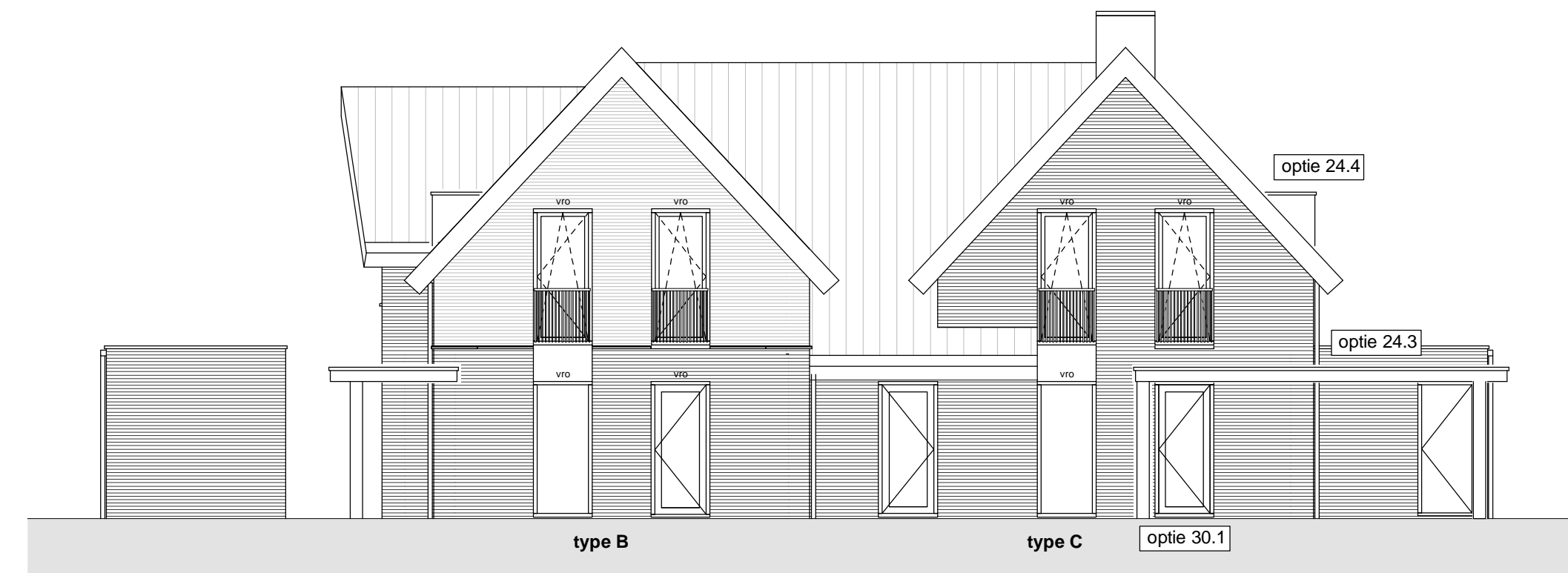
Achtergevel 1 : 100
