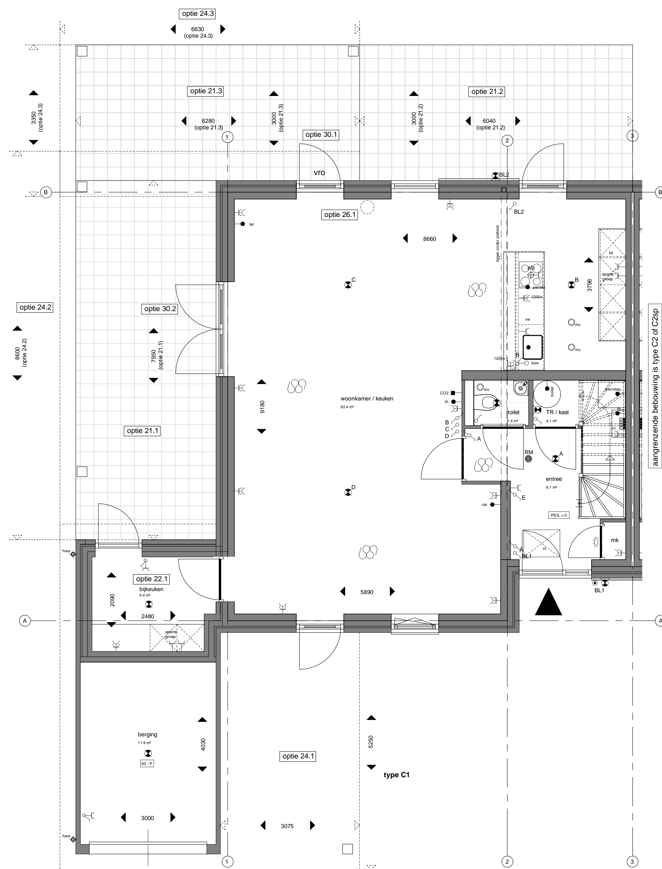
Begane grond type C1 Bouwnummer 5 Bouwnummer gespiegeld 15 1 : 50
