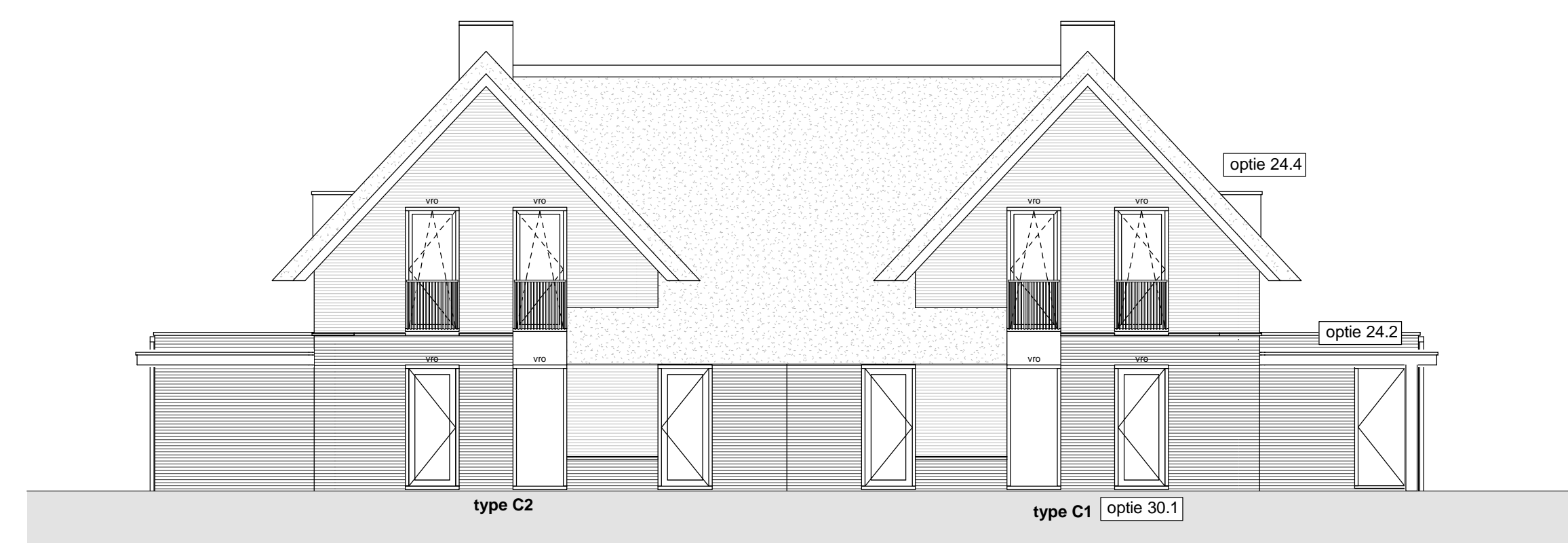
Achtergevel 1 : 100
