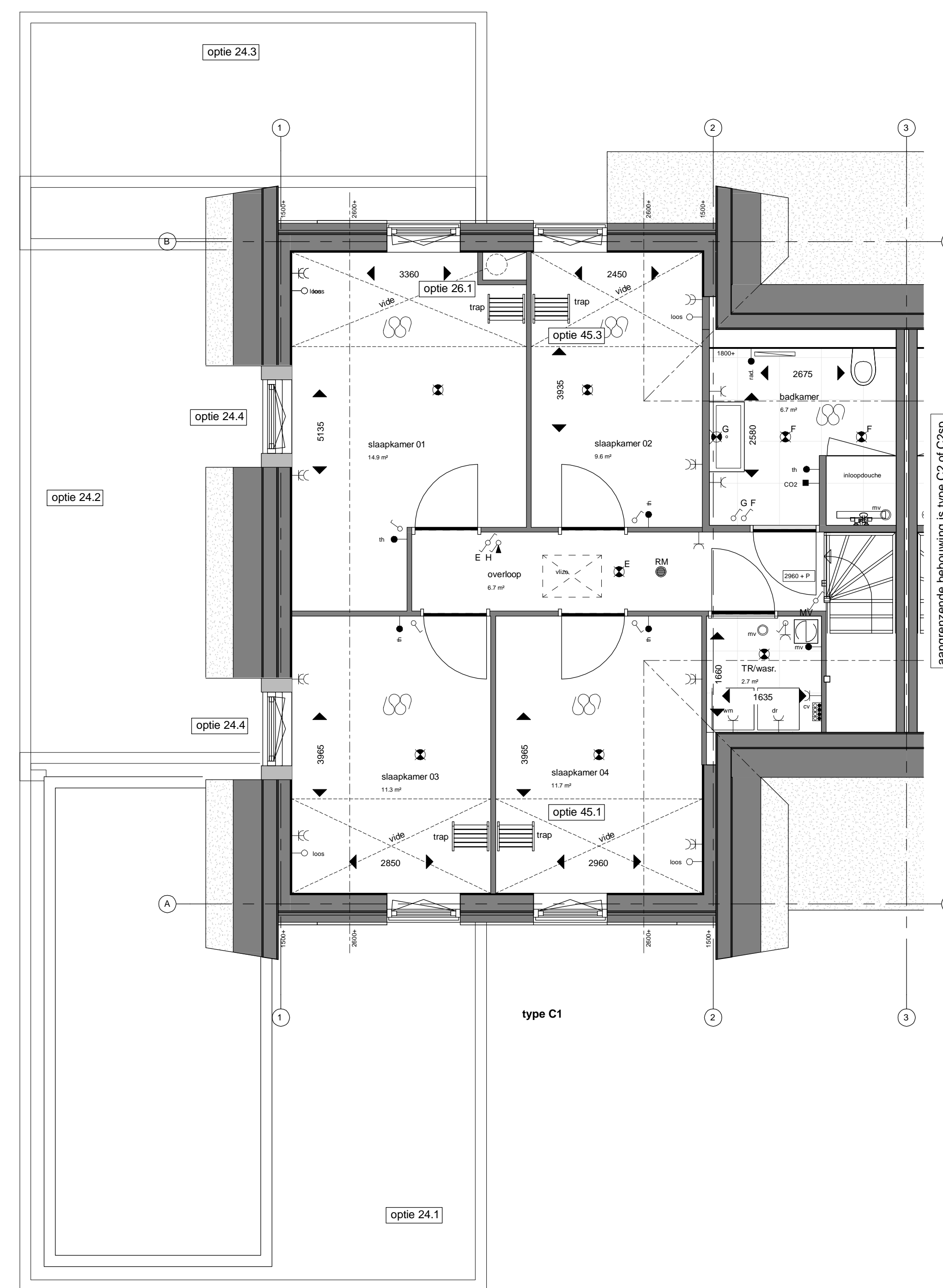
Eerste verdieping type C1 1 : 50
