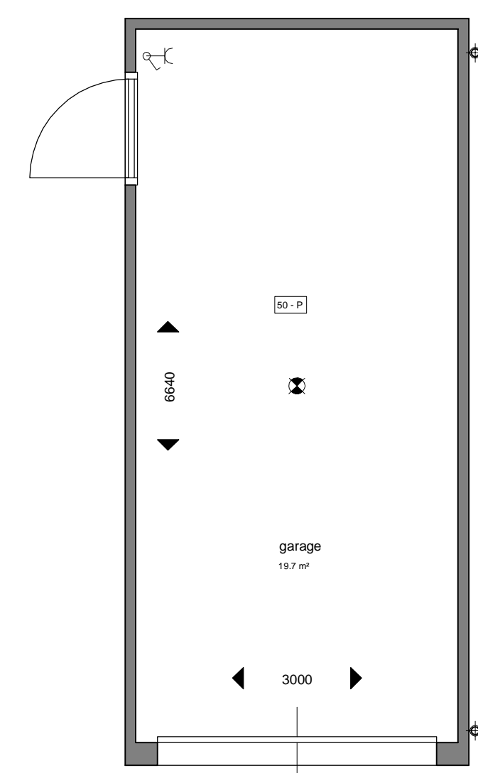
Begane grond type C2 Bouwnummer 4 Bouwnummer gespiegeld 16 1 : 50
