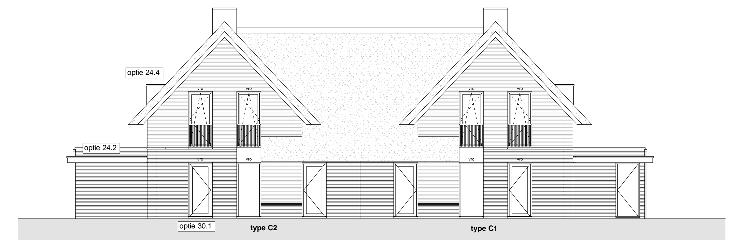
Achtergevel 1 : 100
