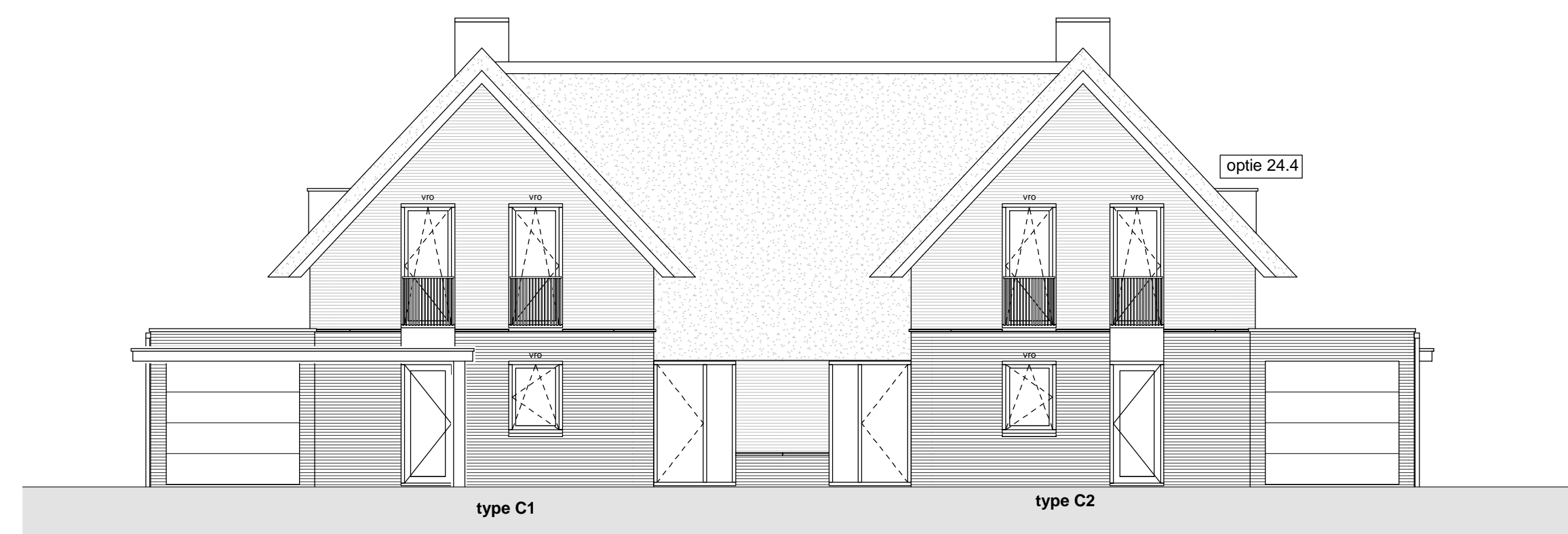
Voorgevel 1 : 100
