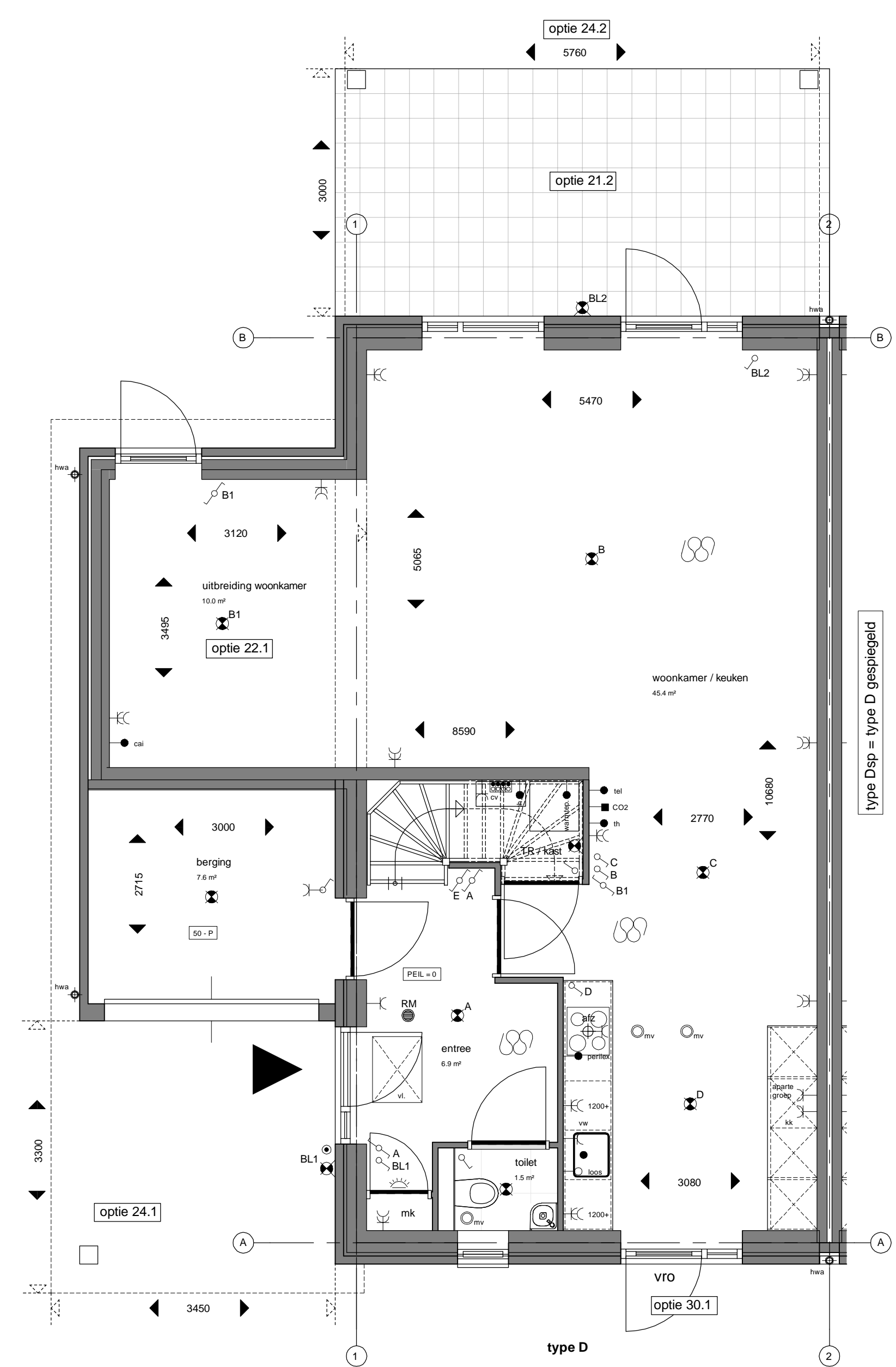
Begane grond type D Bouwnummers 3, 8, 14 en 18 Bouwnummers gespiegeld 2, 7, 13 en 17
