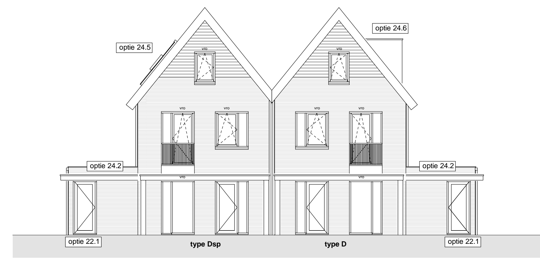
Achtergevel
