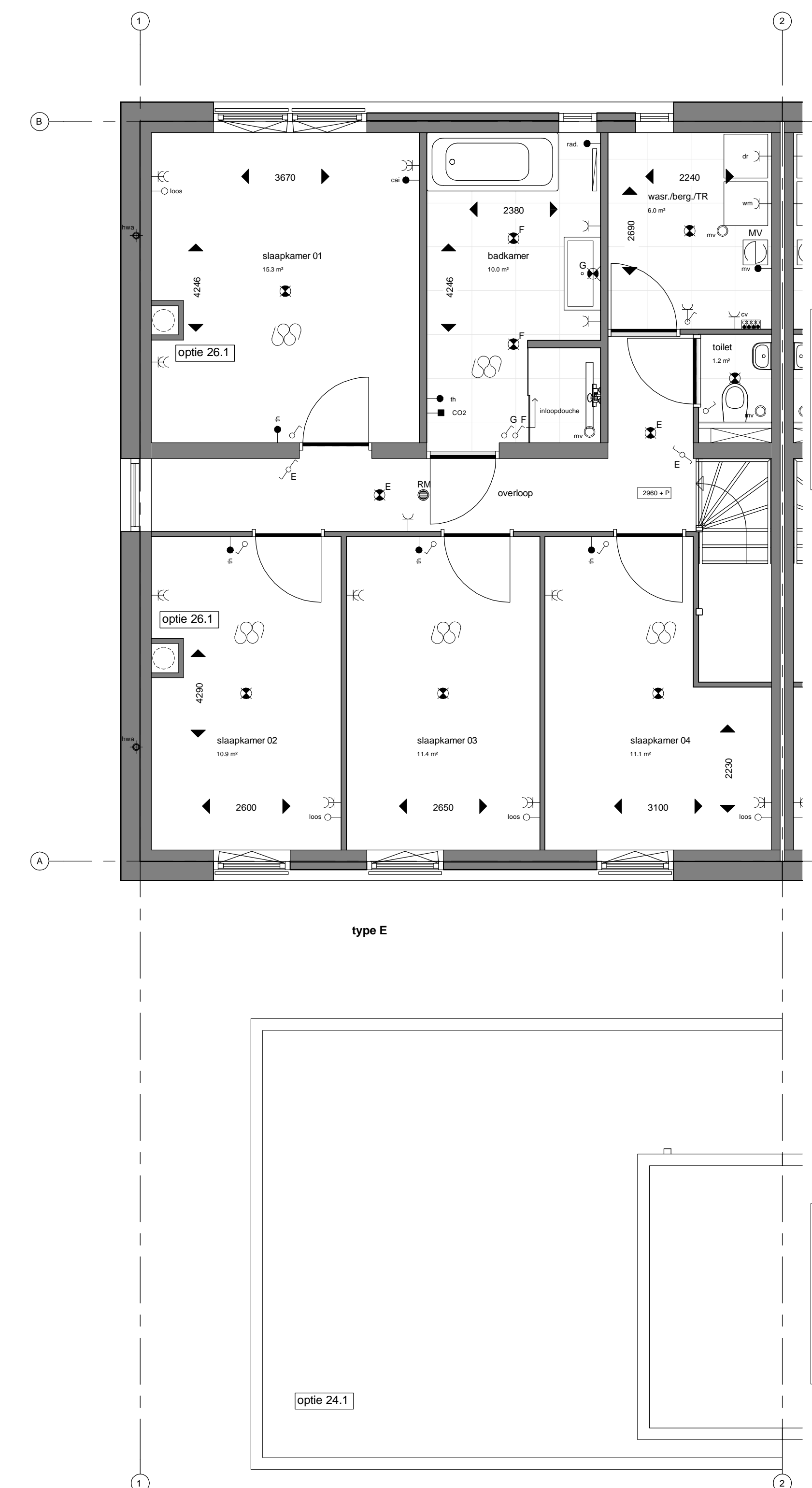
Verdieping type E 1 : 50
