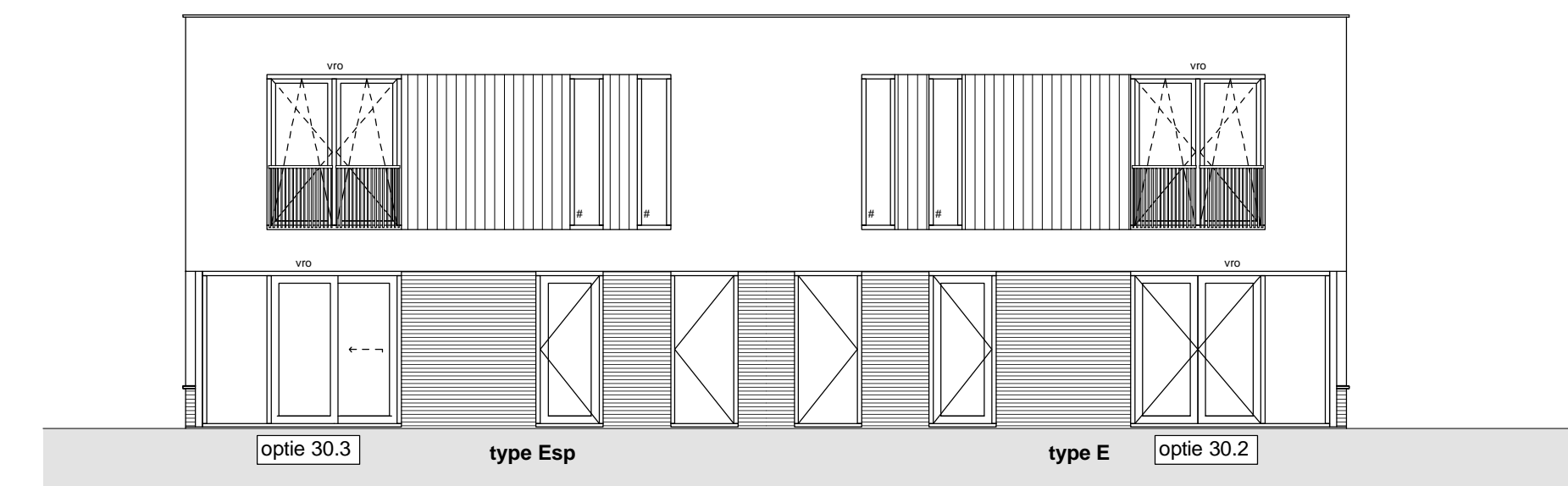
Achtergevel 1 : 100
