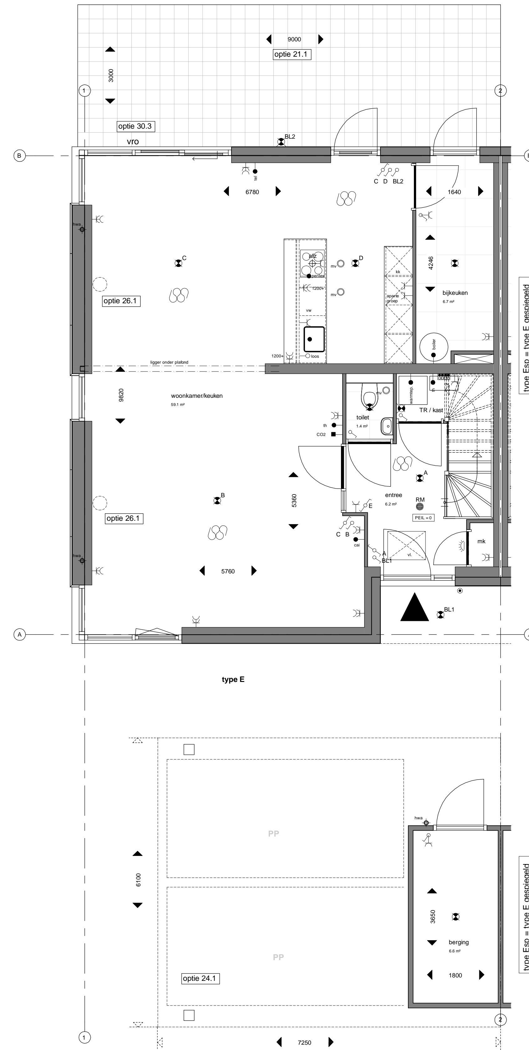
Begane grond type E Bouwnummers 22 en 30 Bouwnummers gespiegeld 21 en 29 1 : 50
