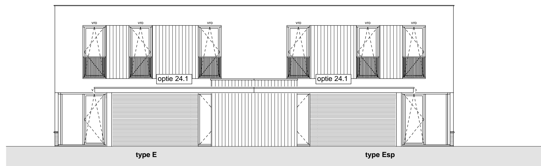
Voorgevel 1 : 100
