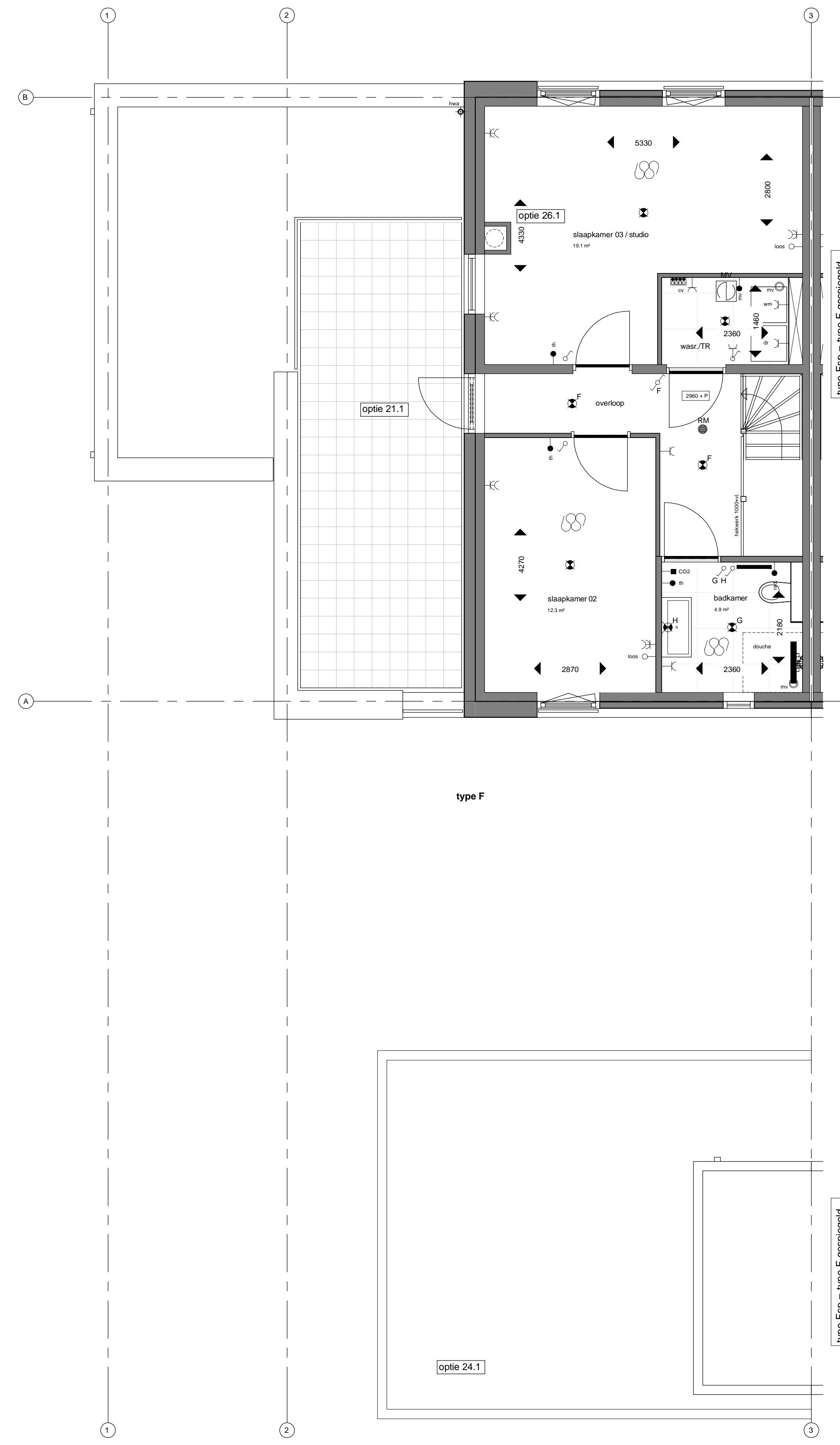
Eerste verdieping type F 1 : 50
