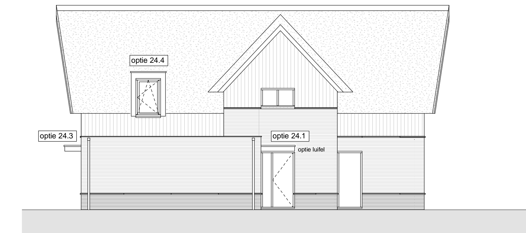
Linkergevel 1 : 100
