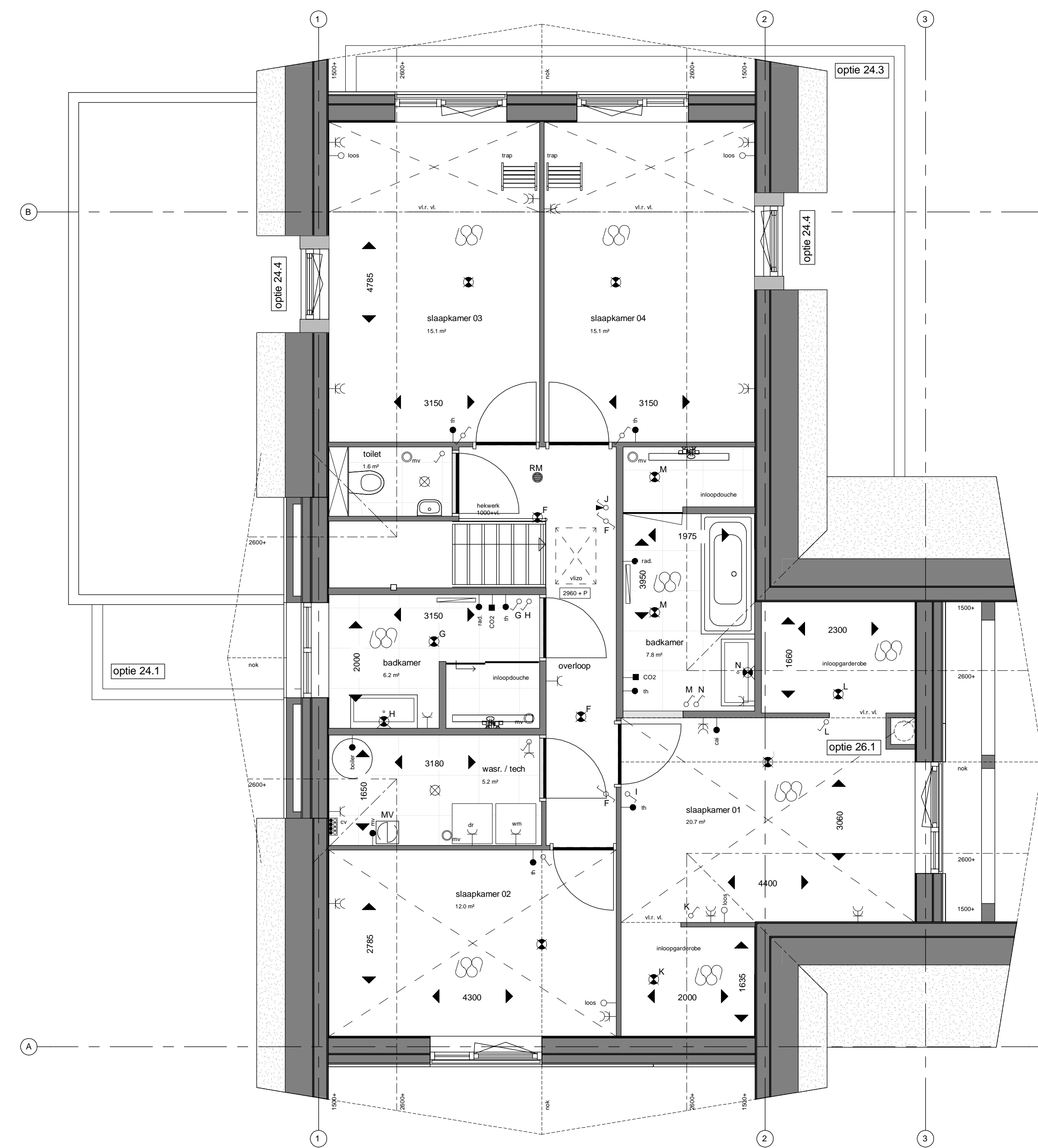
Eerste verdieping type G 1 : 50
