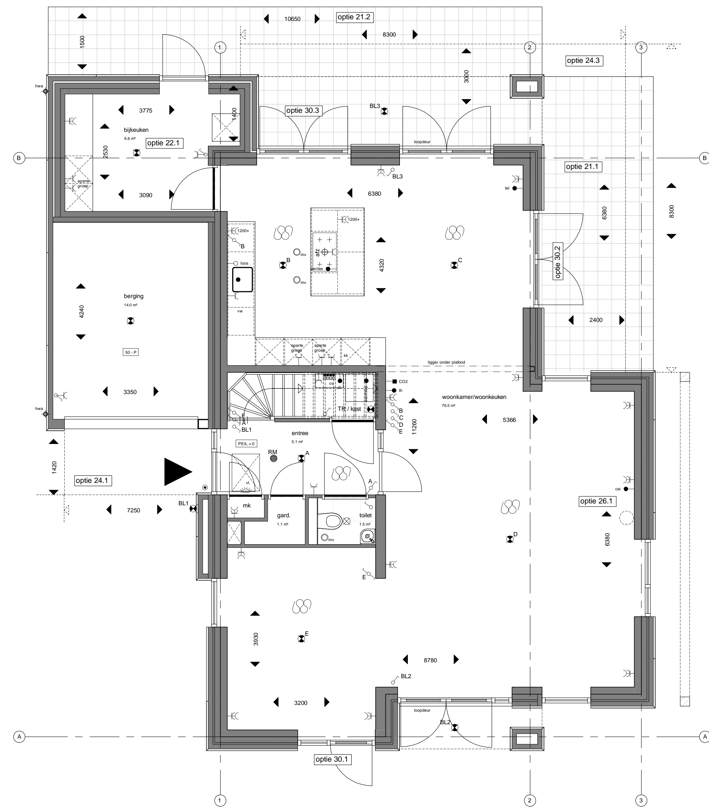
Begane grond type G Bouwnummer 1 Bouwnummer gespiegeld 19 1 : 50
