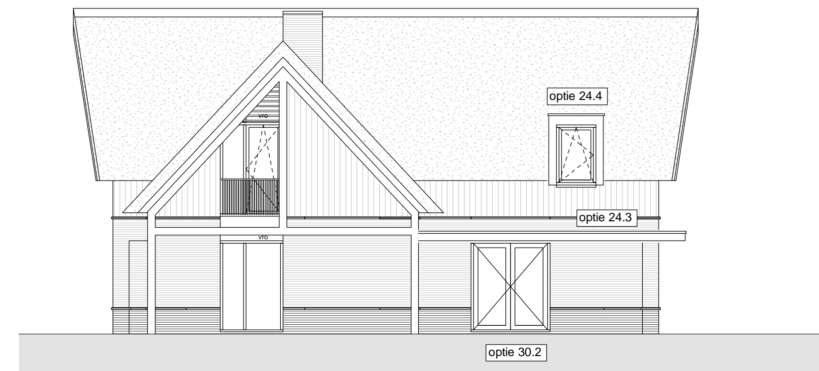
Rechtergevel 1 : 100
