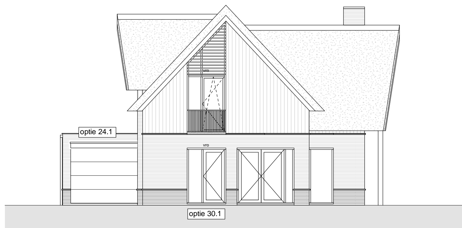
Voorgevel 1 : 100
