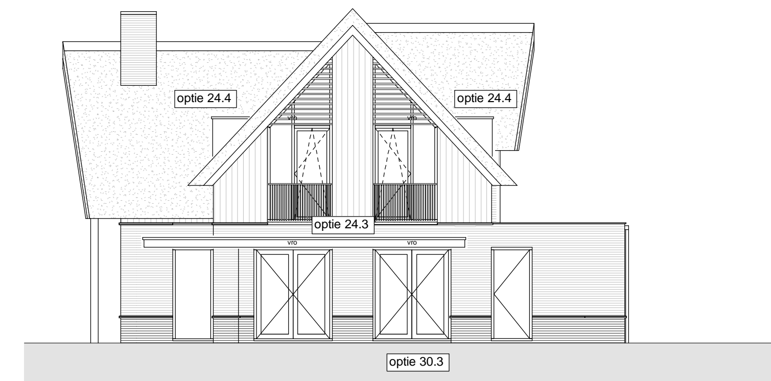
Achtergevel 1 : 100
