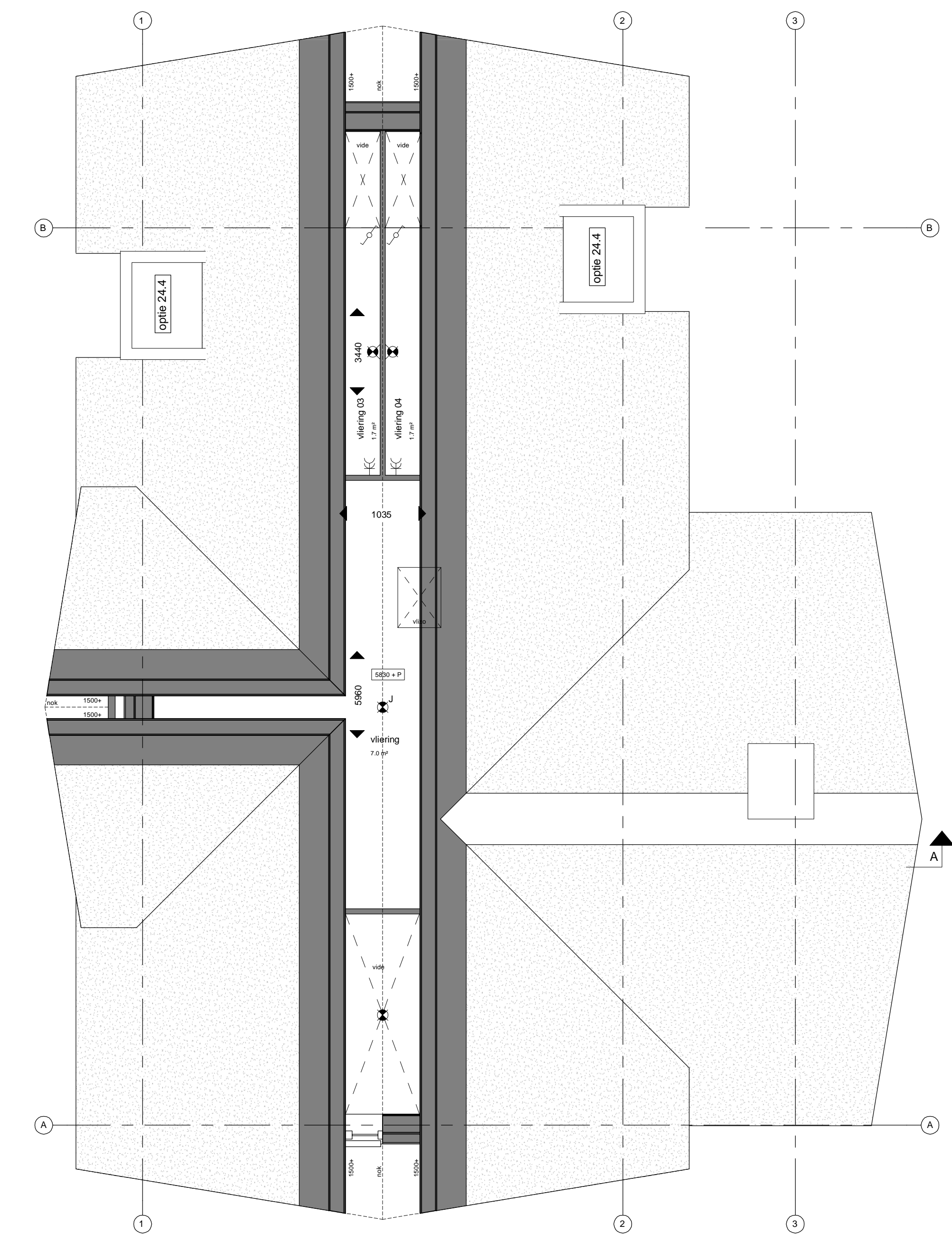
Vliering type G 1 : 50
