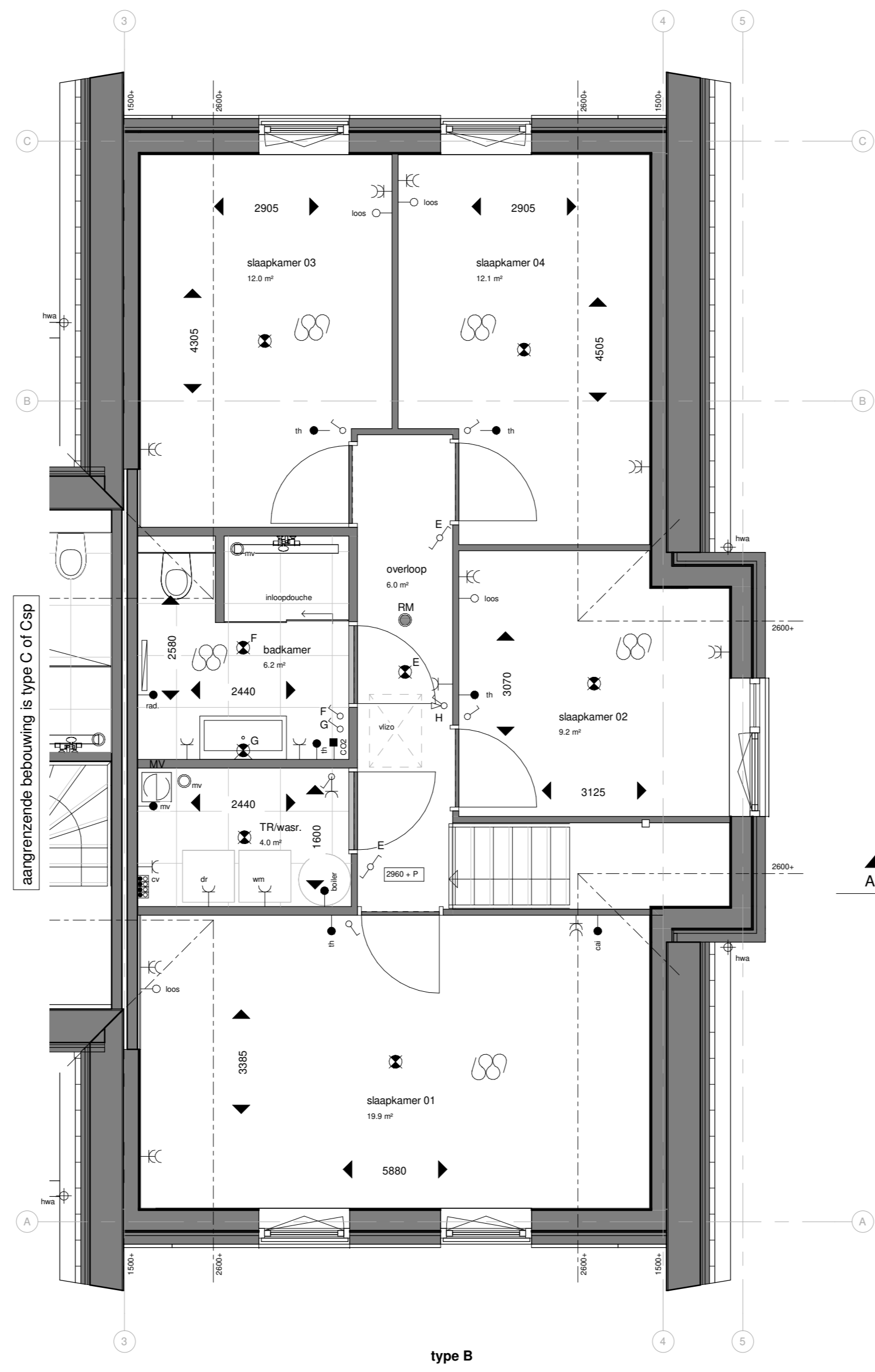
Eerste verdieping type B 1 : 50
