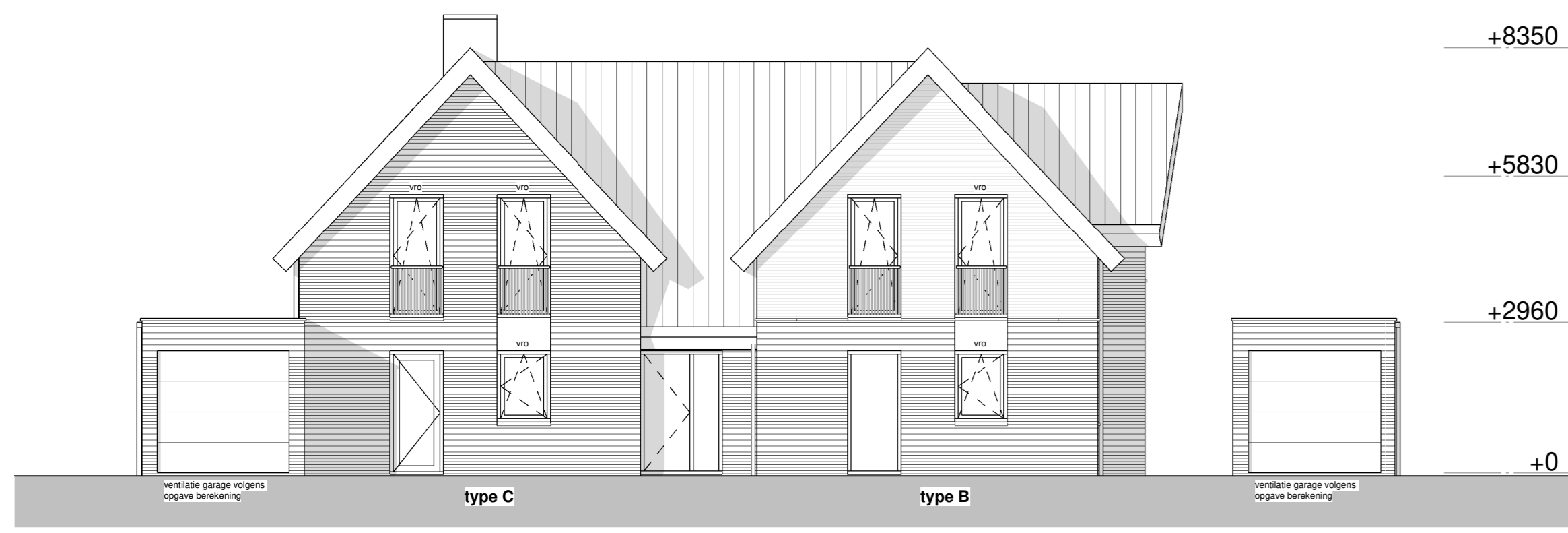
Voorgevel 1 : 100
