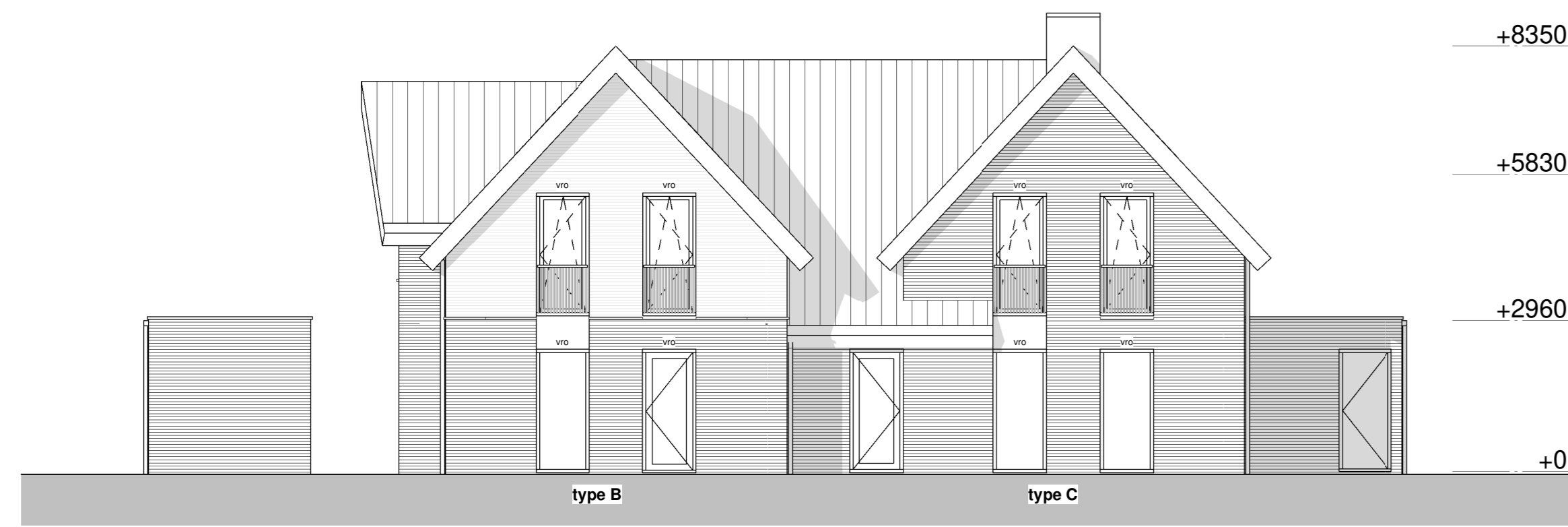
Achtergevel 1 : 100
