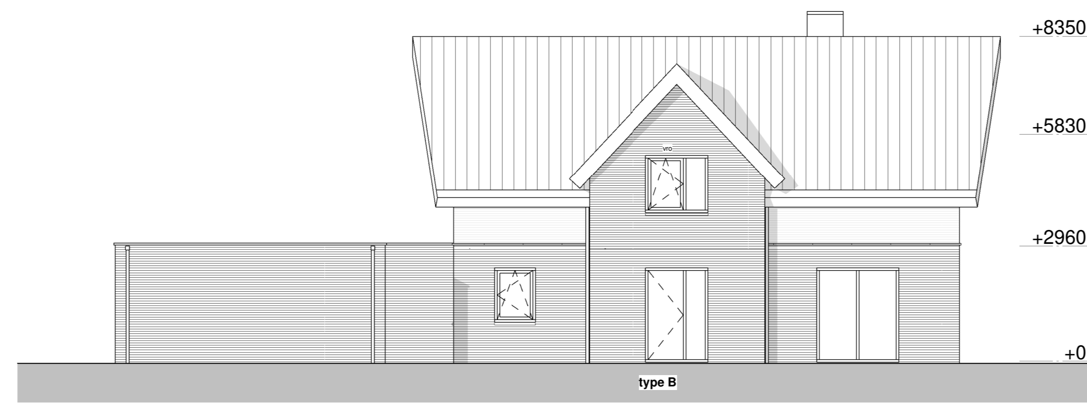
Rechtergevel 1 : 100
