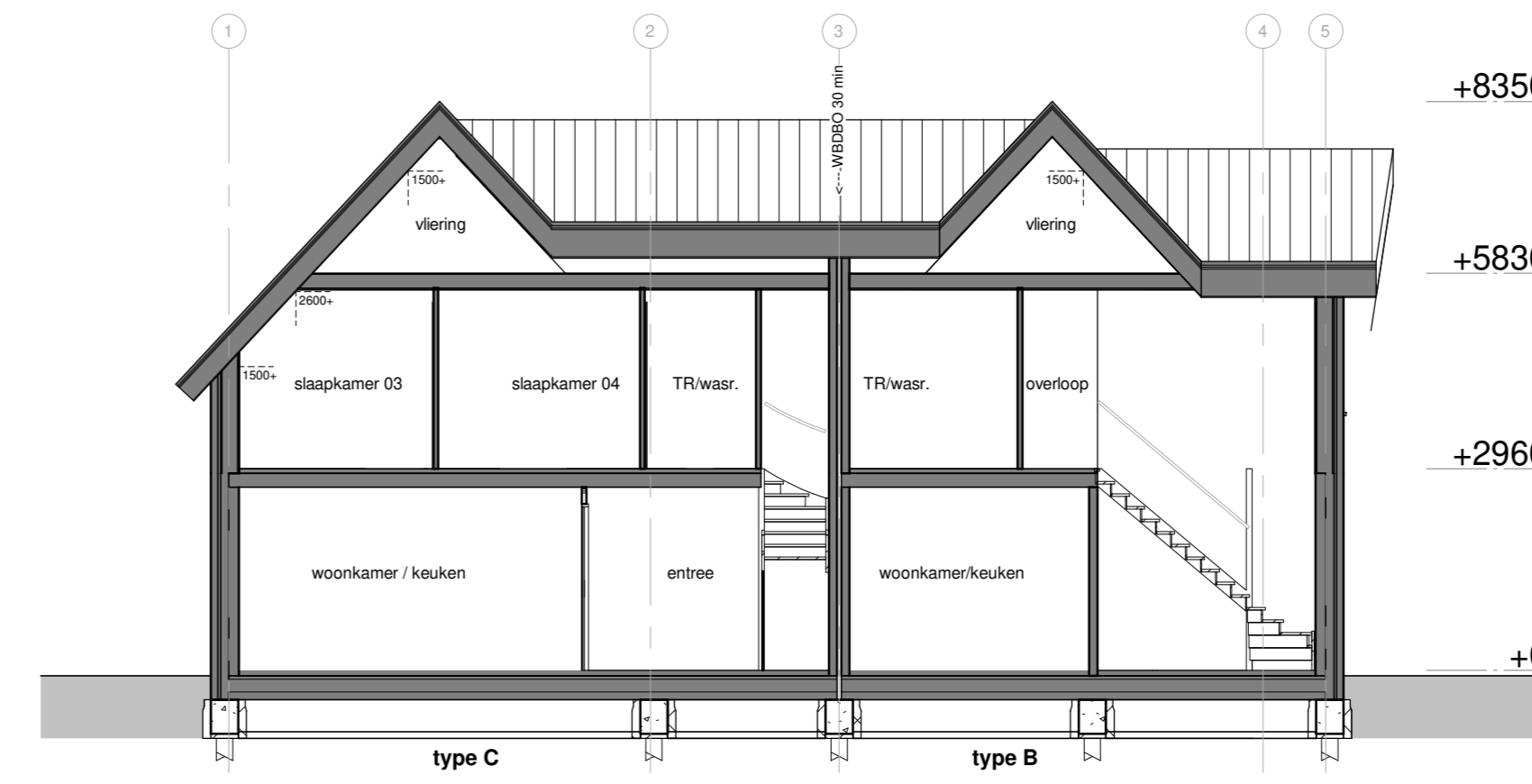
Doorsnede A-A 1 : 100
