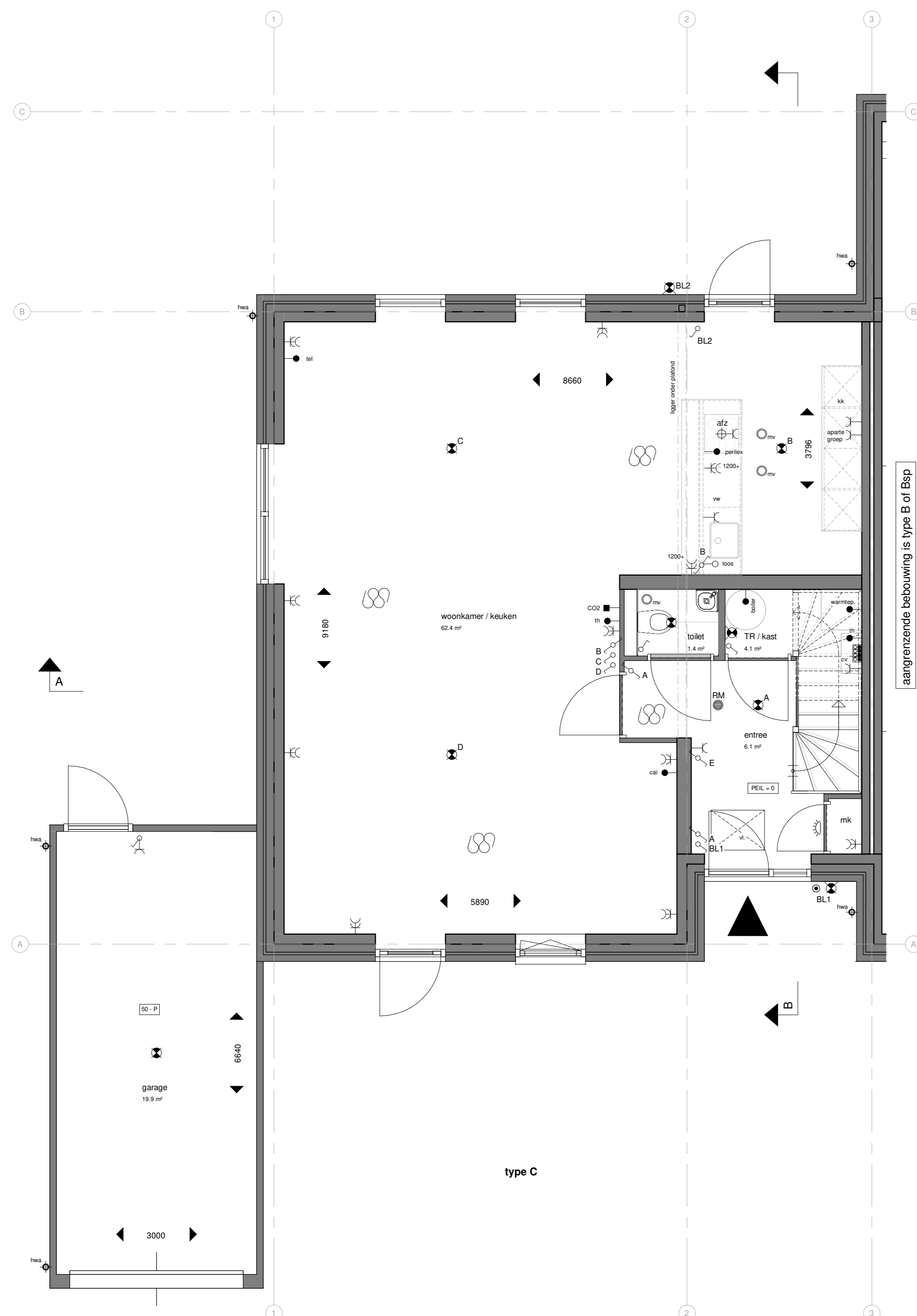
Begane grond type C Bouwnummer 12 Bouwnummer gespiegeld 9 1 : 50
