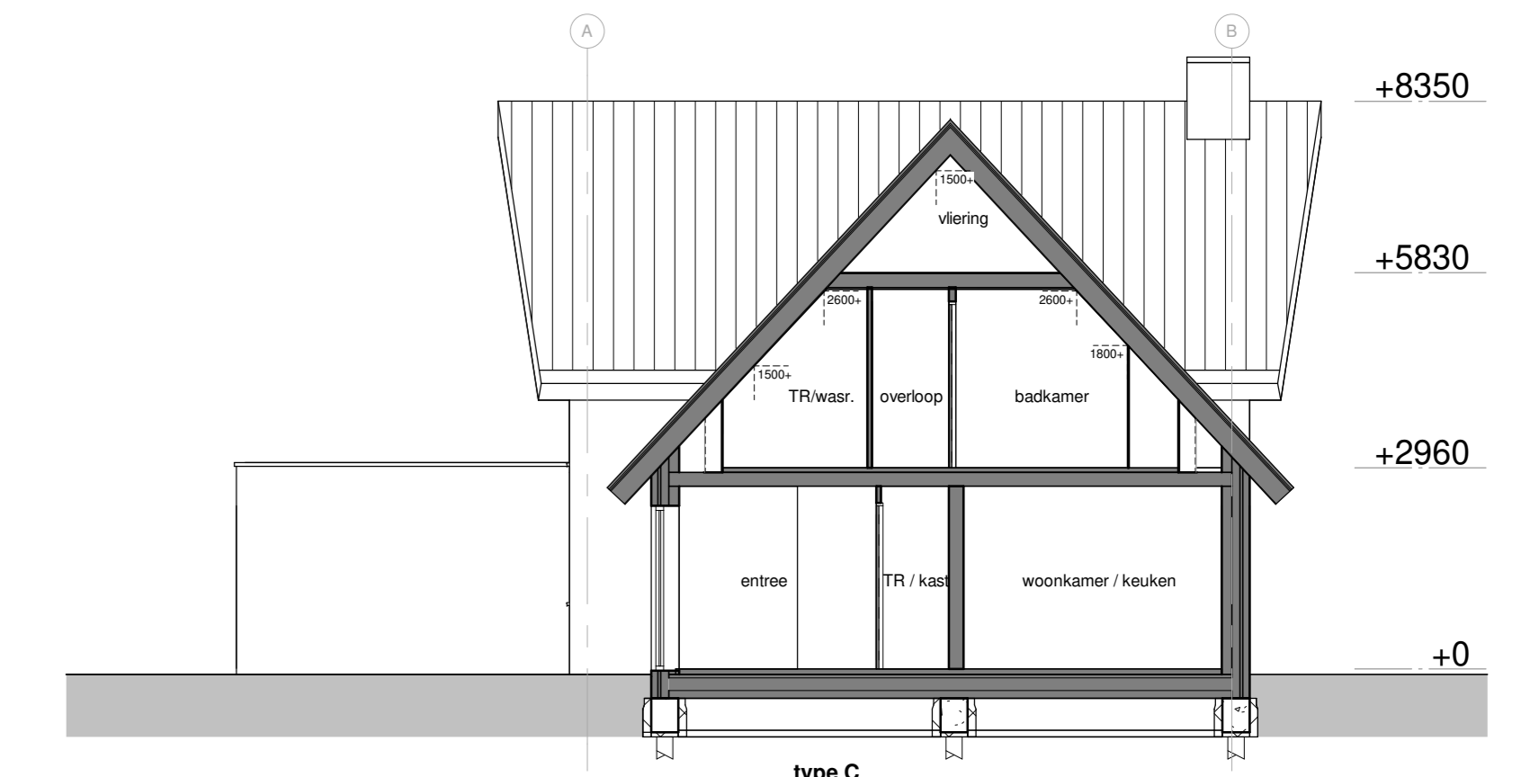
Doorsnede B-B
