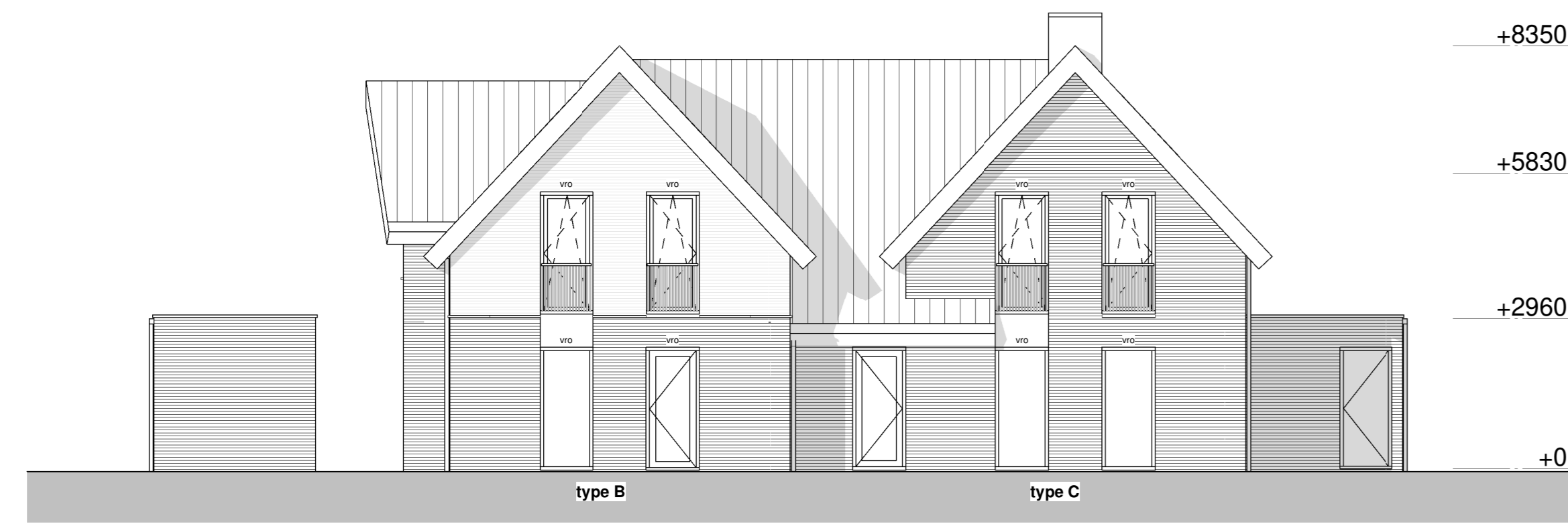
Achtergevel
