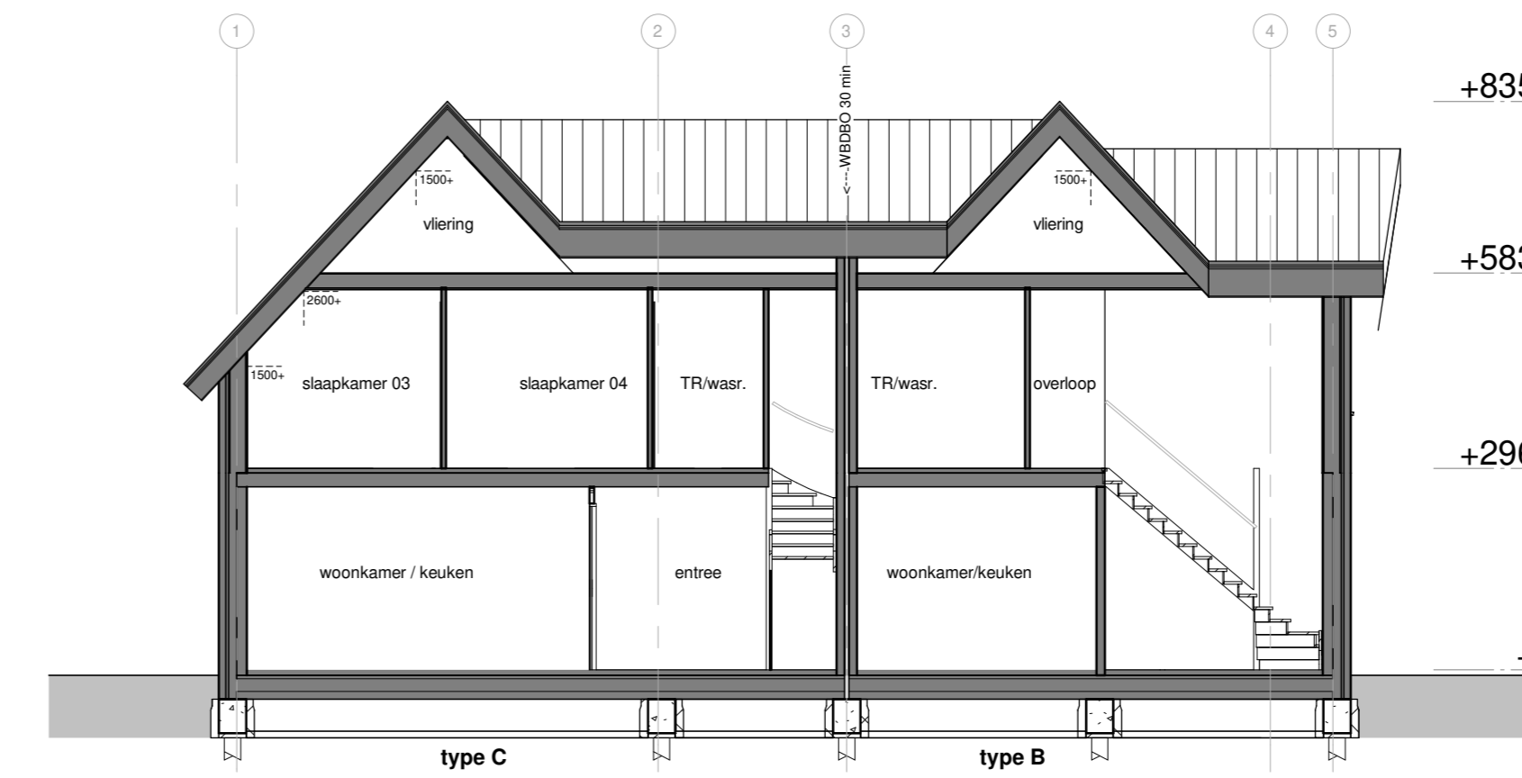
Doorsnede A-A
